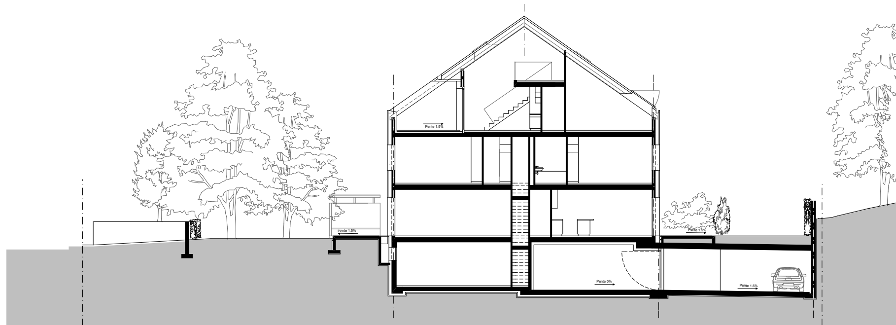
COUPE A-A
