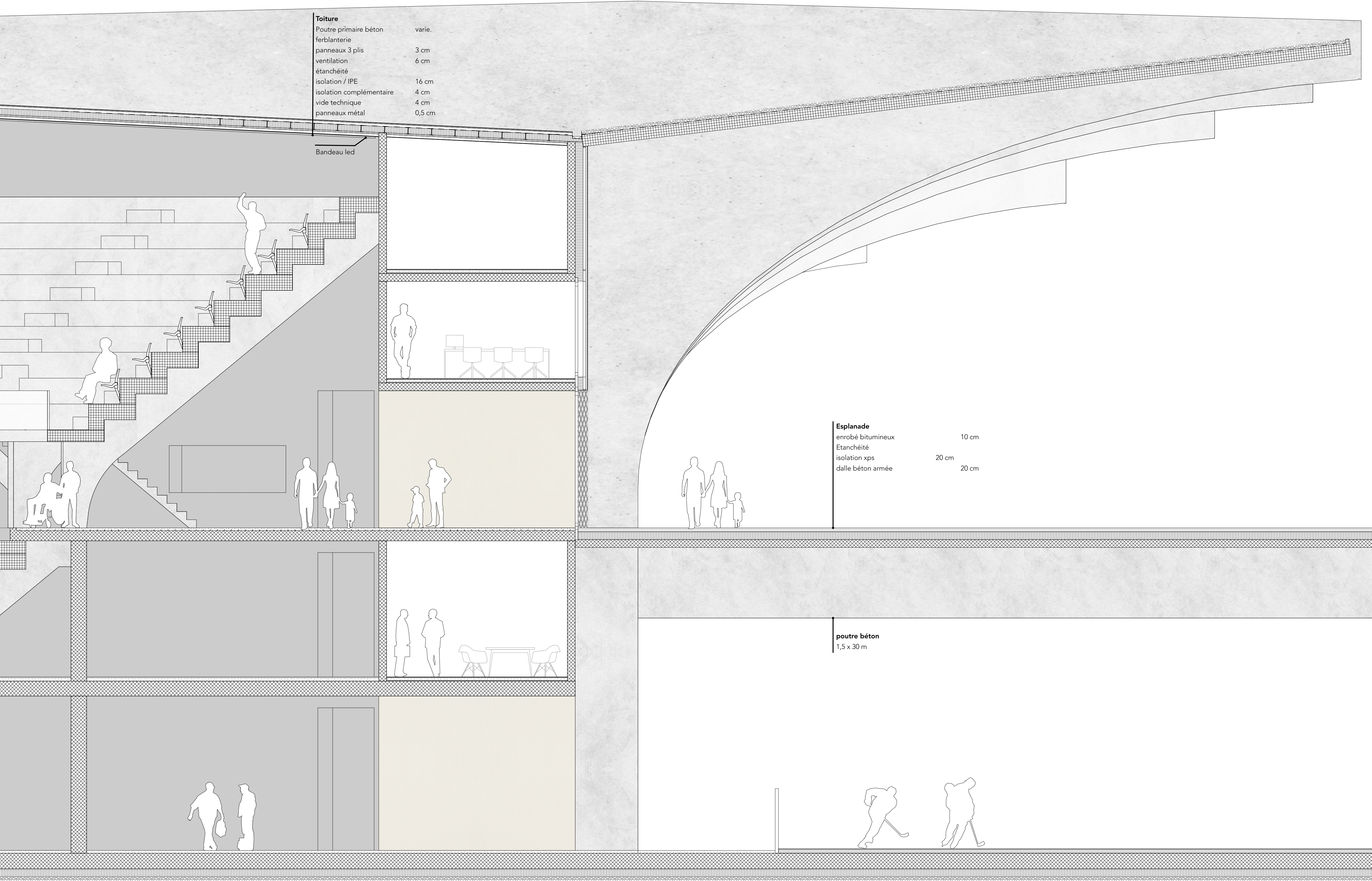
Détail de la coupe A 1/50
