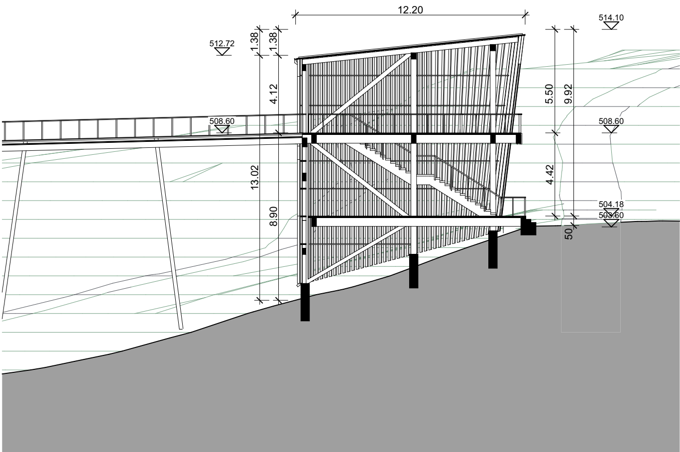
Längsschnitt S - S
