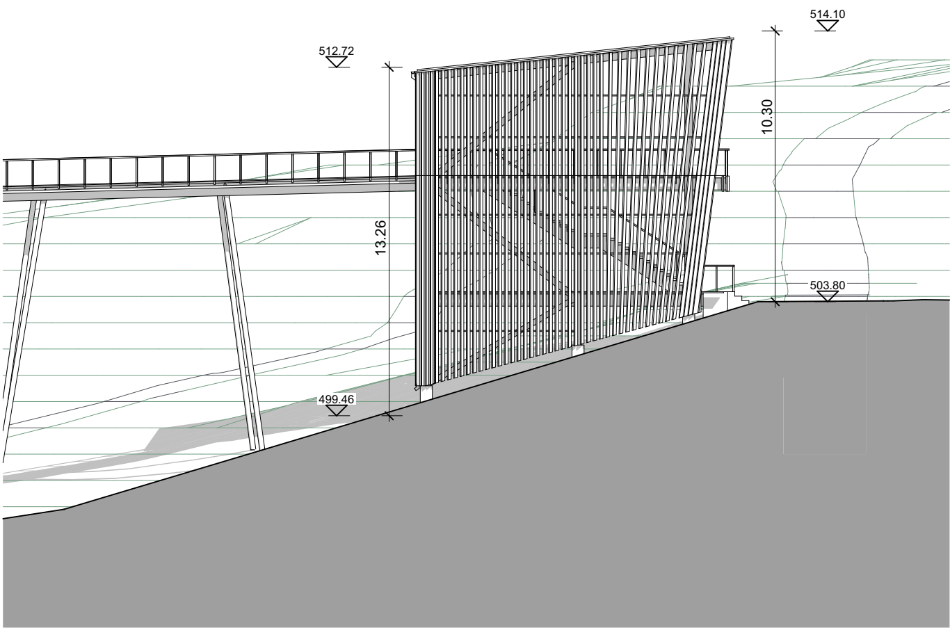
Ansicht West
