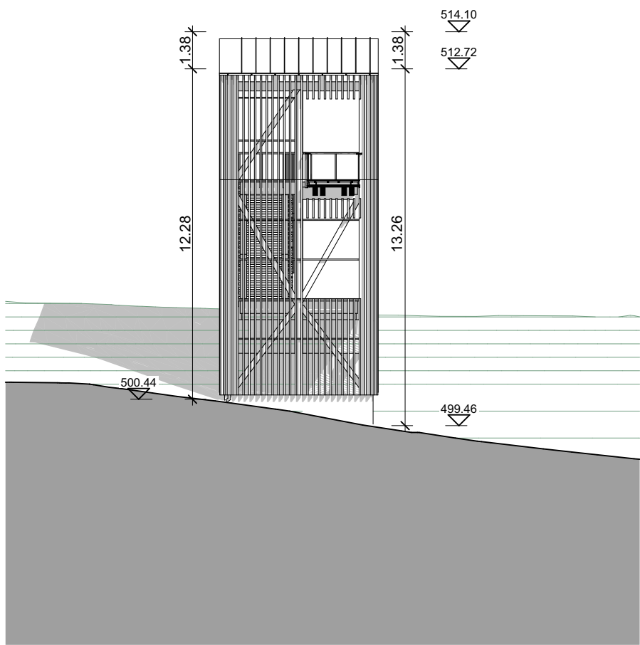
Ansicht Nord
