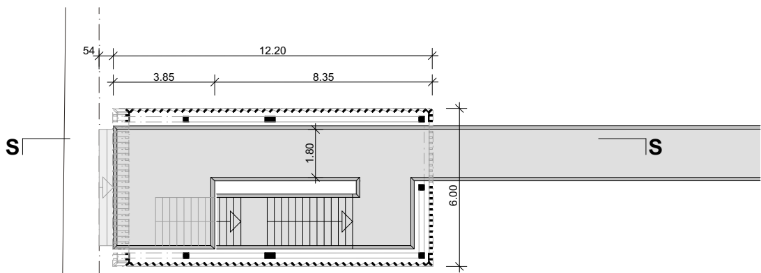
Grundriss
