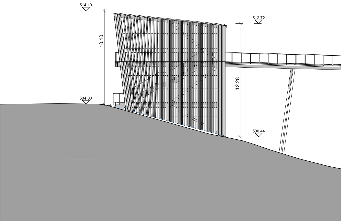
Ansicht Ost
