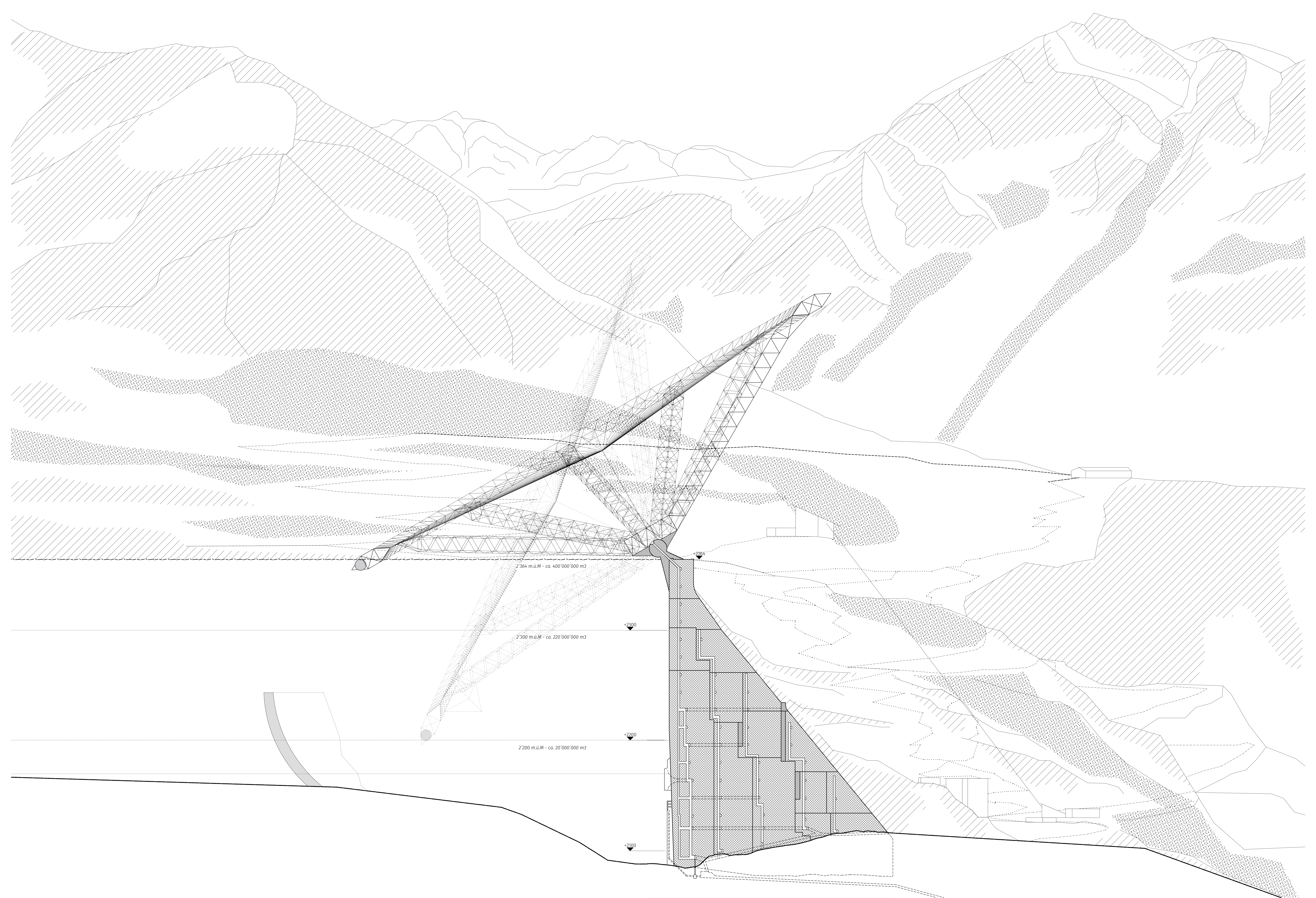
Schnitt - 1 : 1000
