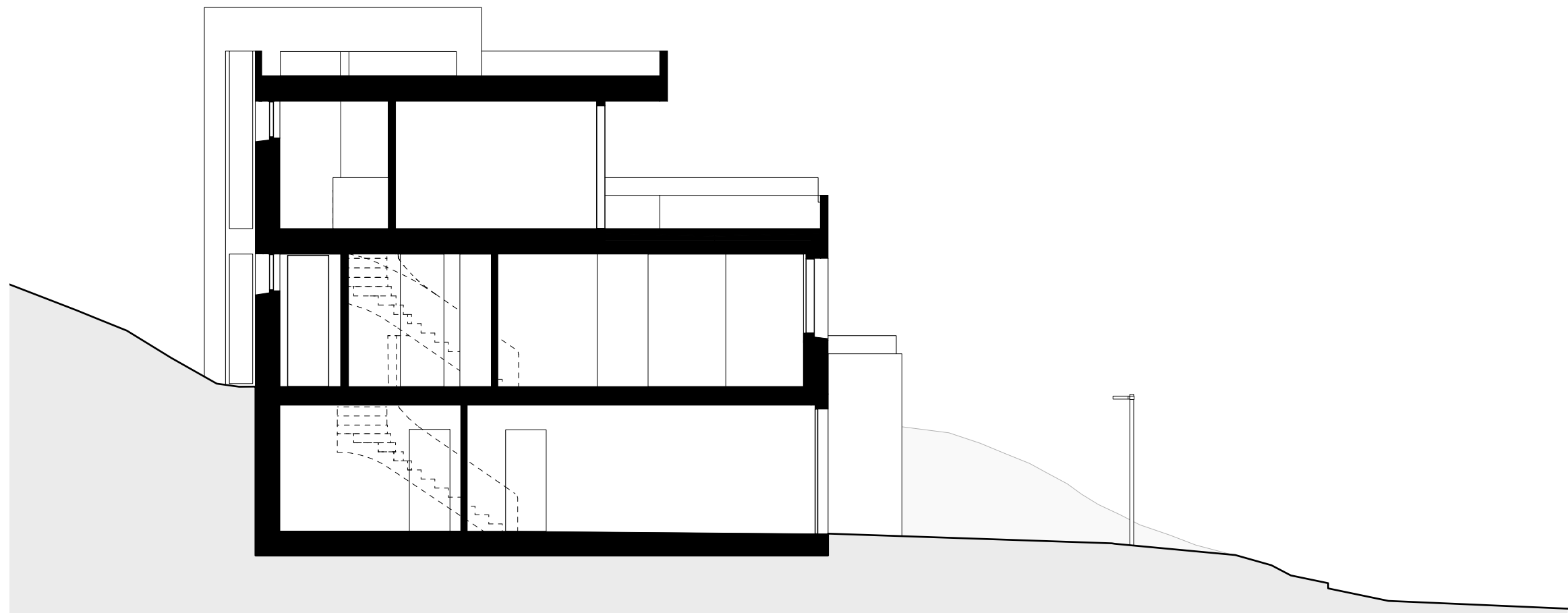
Querschnitt 1 1:100
