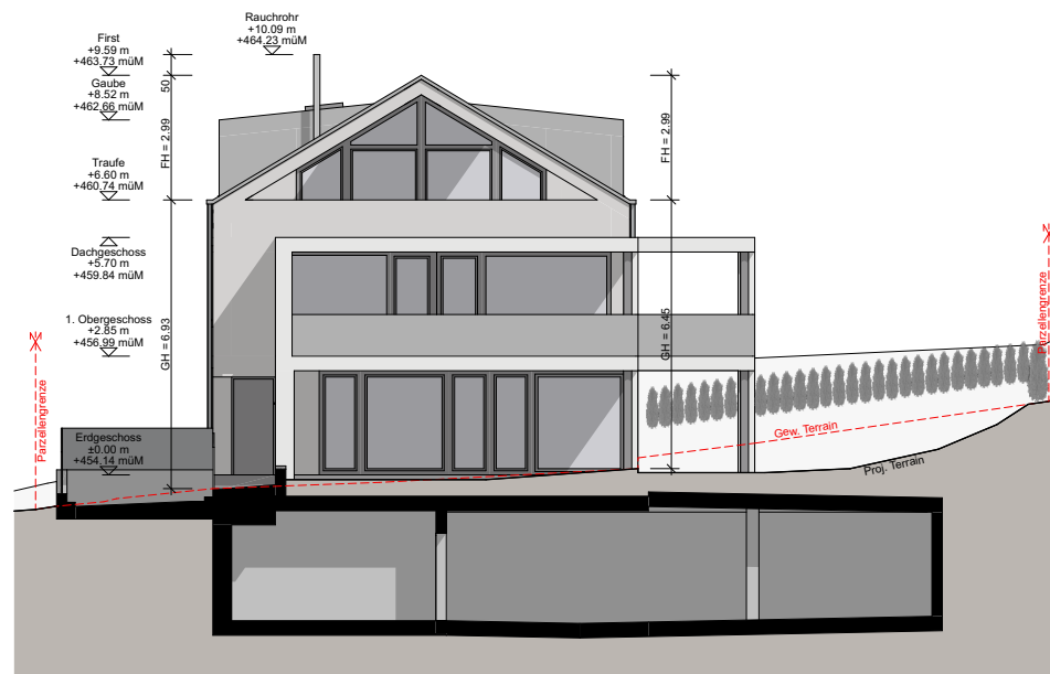
Ansicht West
