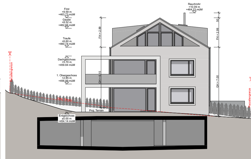
Ansicht Ost
