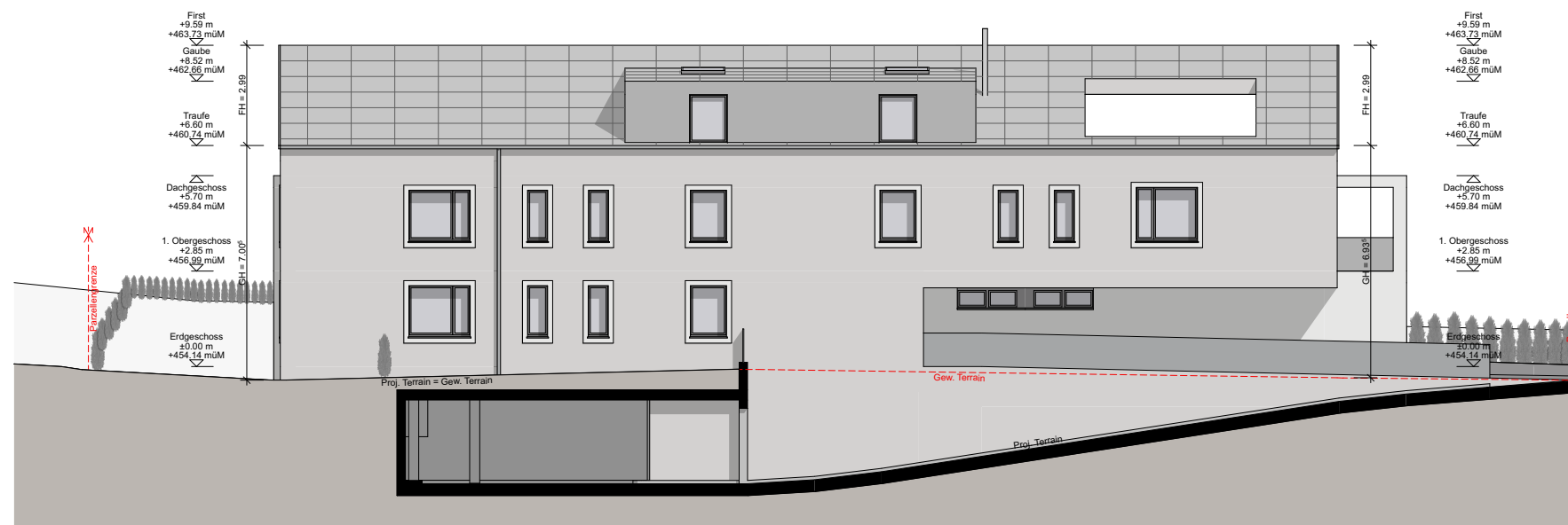
Ansicht Nord
