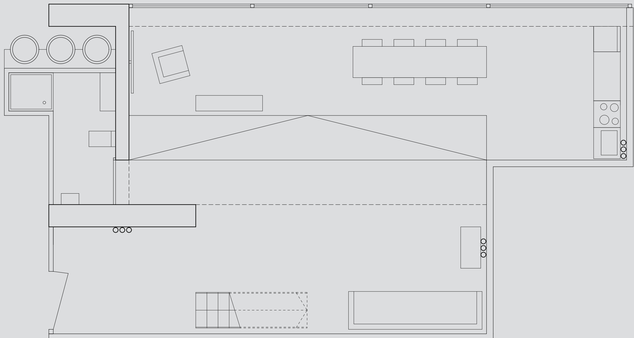
Wohnungsgrundriss EG 1 : 50
