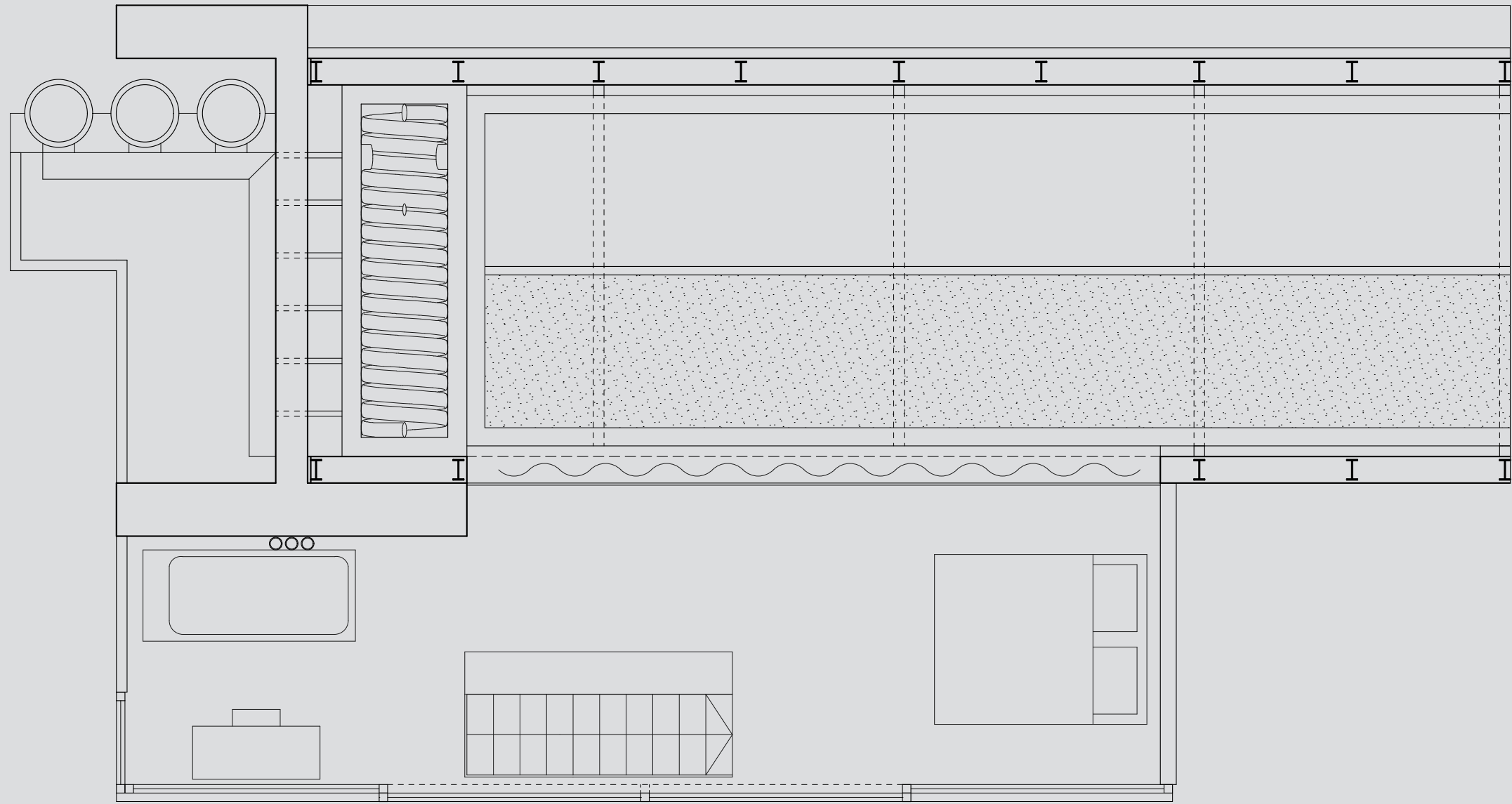
Wohnungsgrundriss OG 1 : 50
