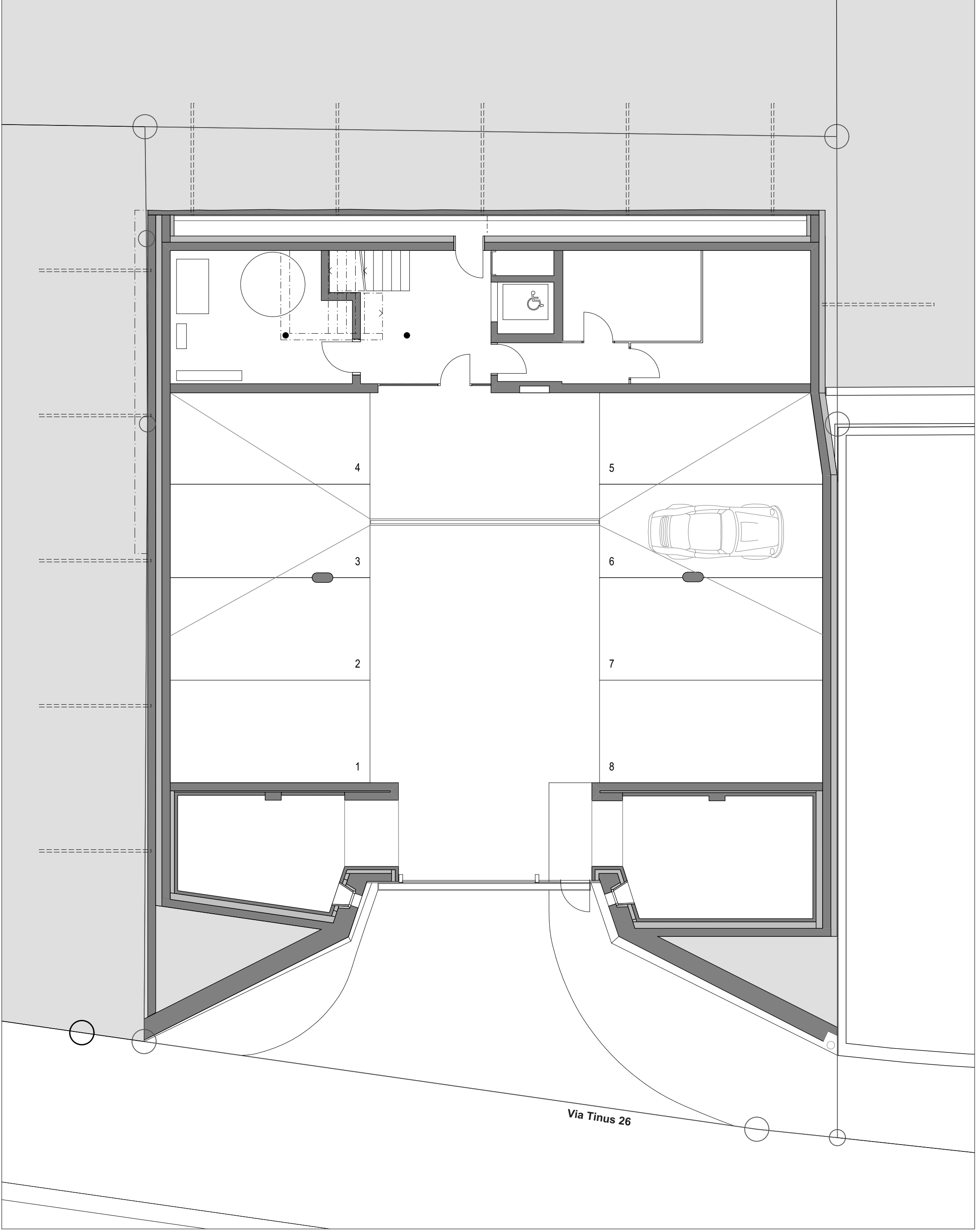
GRUNDRISS UNTERGESCHOSS
