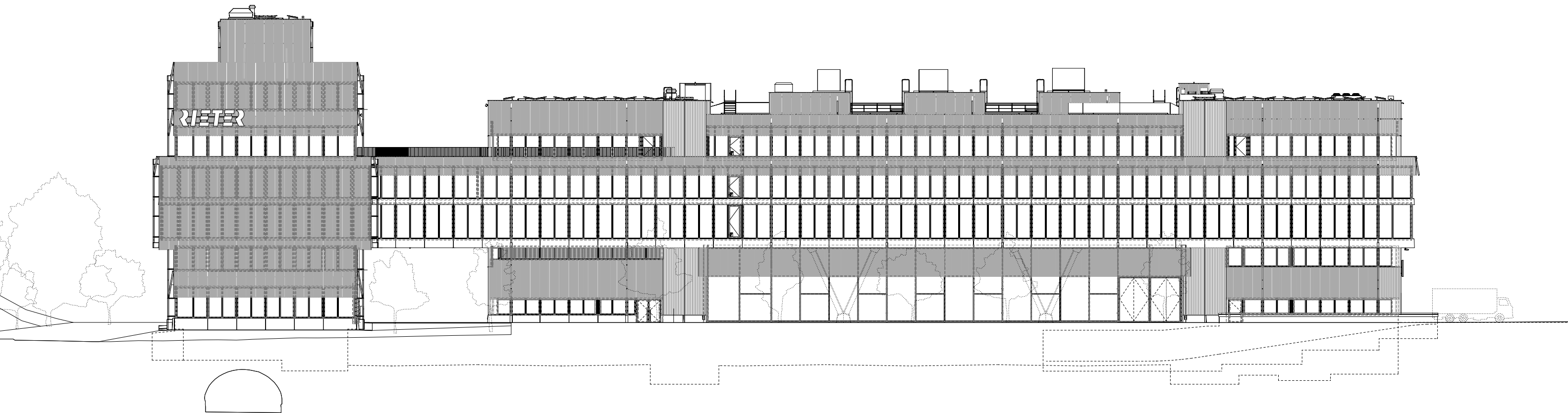
ANSICHT SÜD HQ/TC
