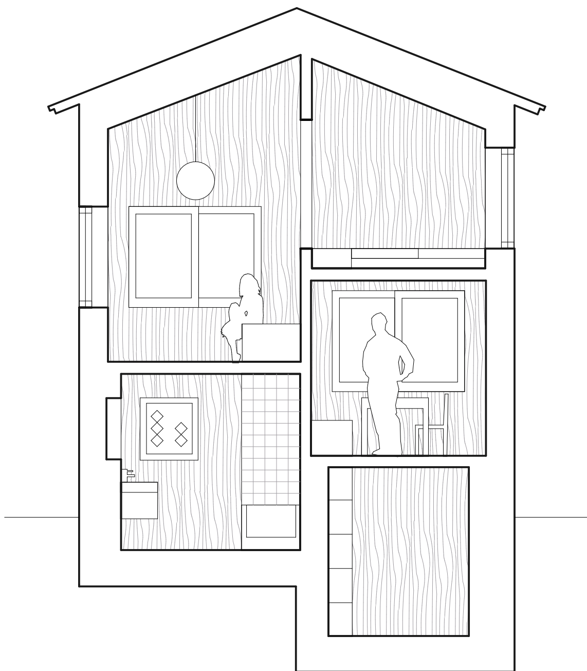
coupe 1:50
