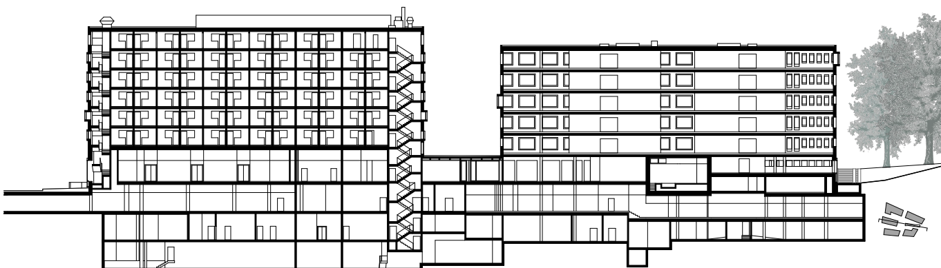
Bleiche Schaffhausen - Schnitte Pfister Schiess Tropeano + Partner Architekten AG
