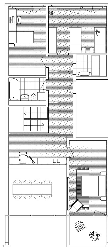
GARTENMAISONETTE 1.OG
