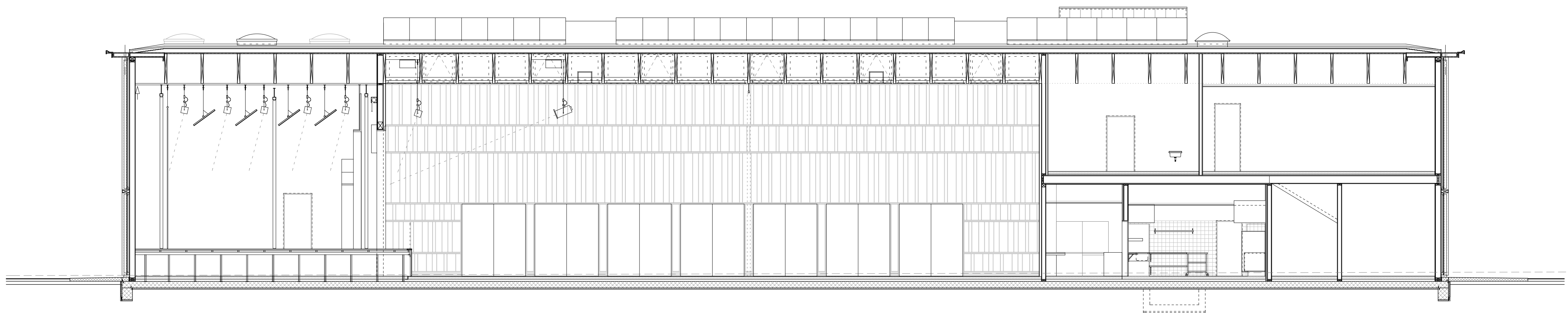
Längsschnitt G - G
