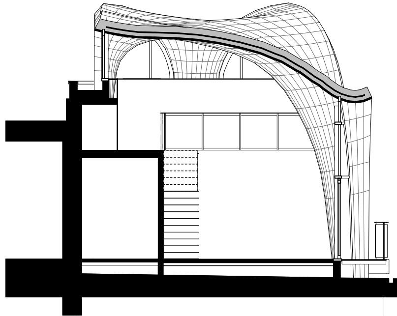
Schnitt Quer M 1:100
