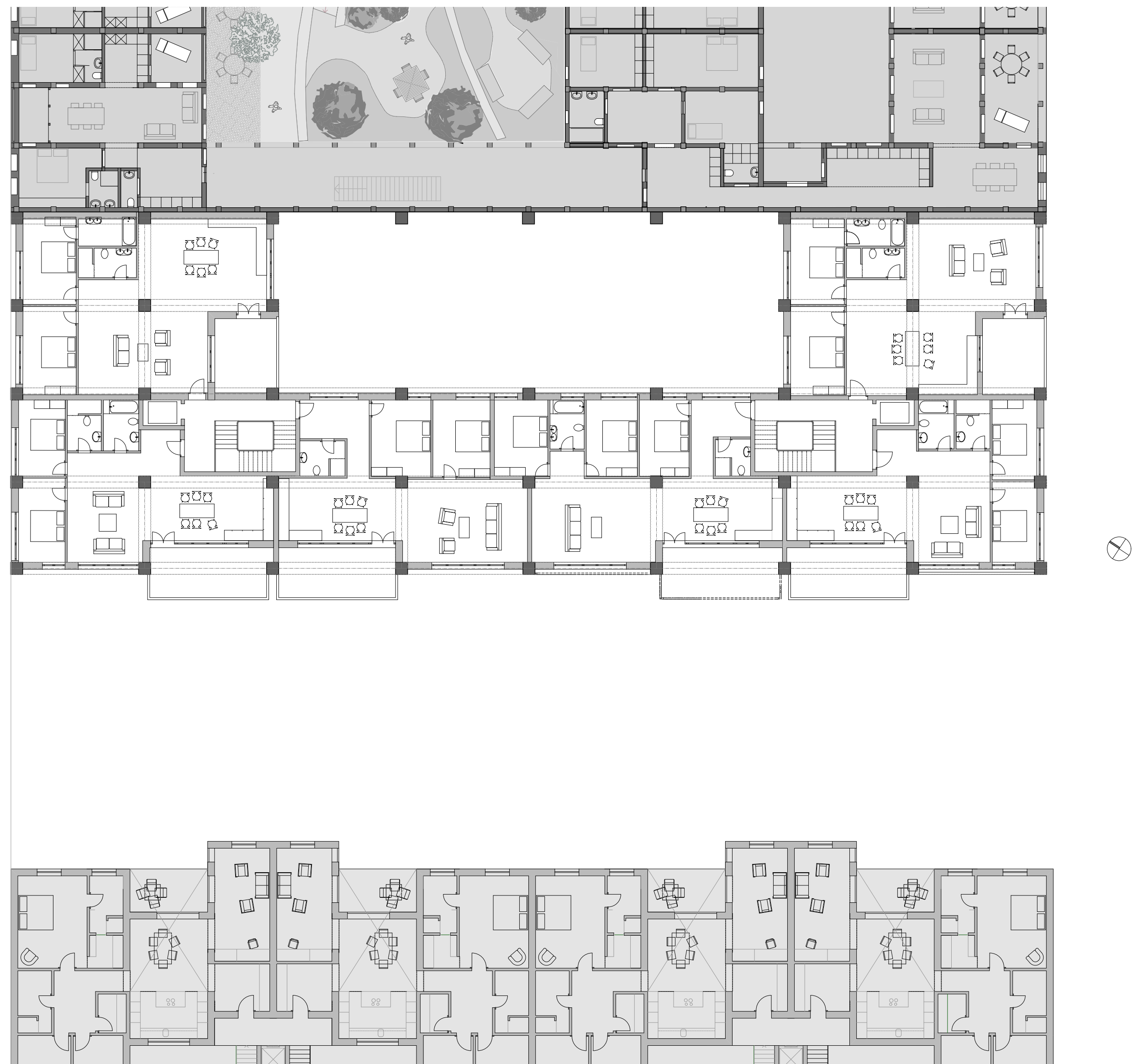
1. - 3. Obergeschoss 1:200
