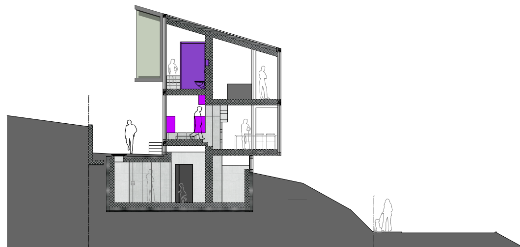
Quer-Schnitt 2 Mst.: 1:200
