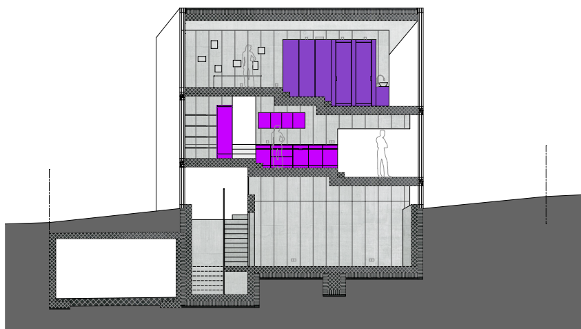
Längs-Schnitt 2 Mst.: 1:200
