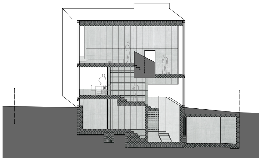
Längs-Schnitt 1 Mst.: 1:200
