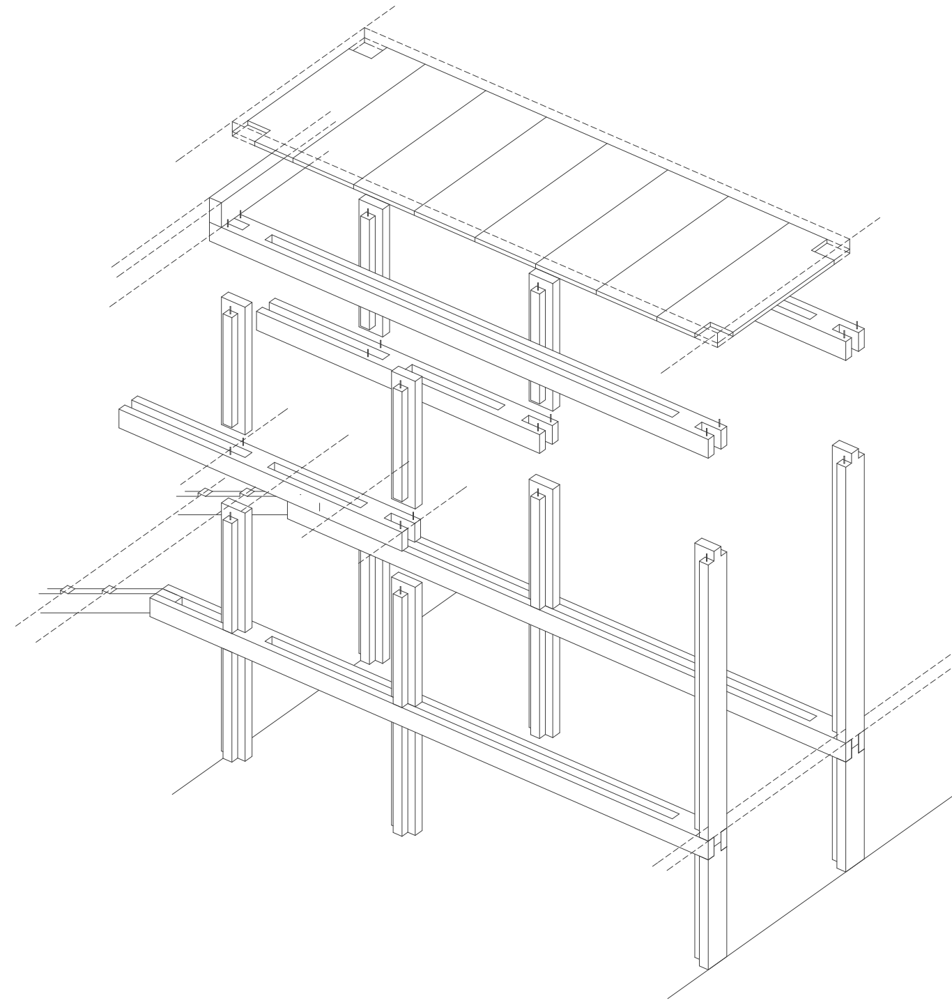
Tragwerksschema
