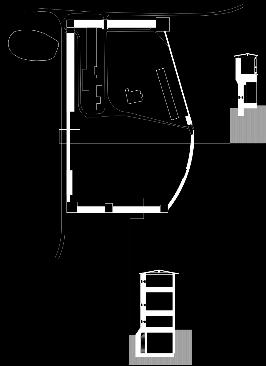
Nowgorod-Jurjew Kloster Maueranalyse
