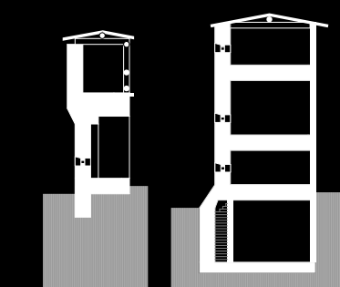
Dreieinigkeits- Sergius- Lawra Kloster: - Mauer mit „Brückenverbindungen“
