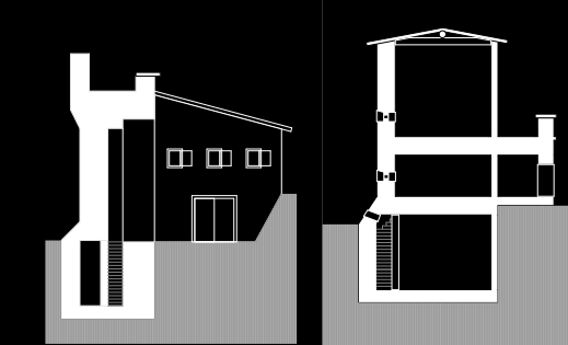
Neujungfrauen Kloster - Schiesschartennische - Anschluss an Schwarzpulver Kammer
