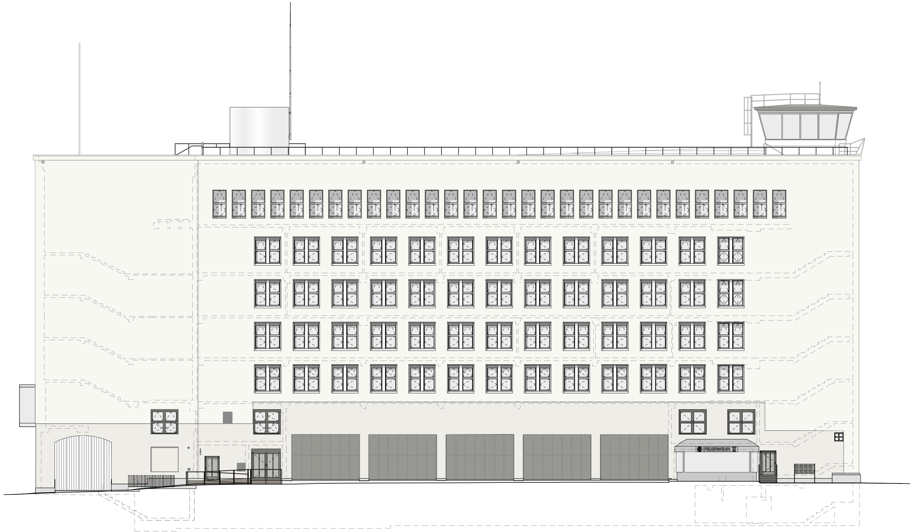
THF - Ansicht Süd
