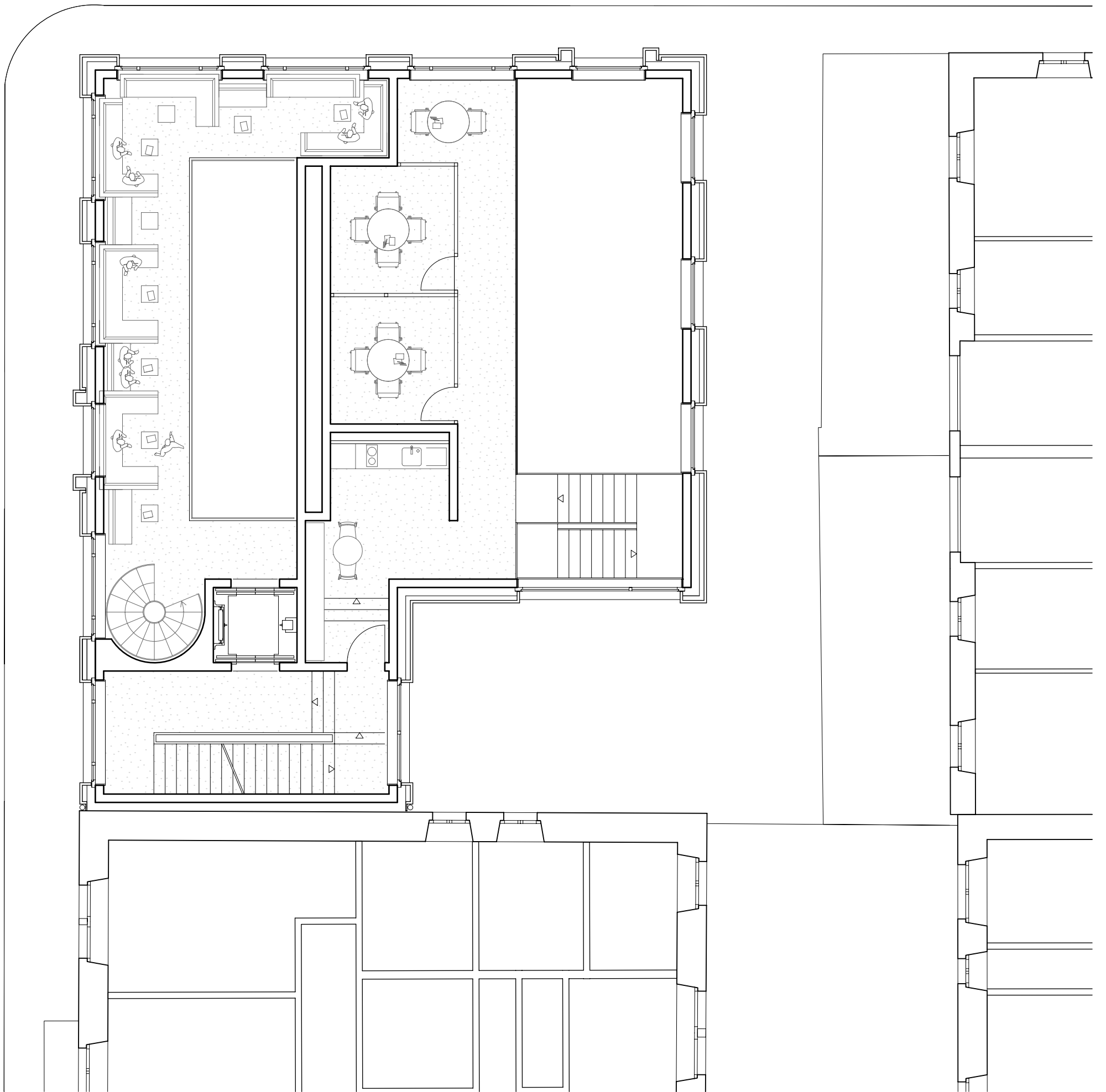
Grundriss 1. OG 1:100
