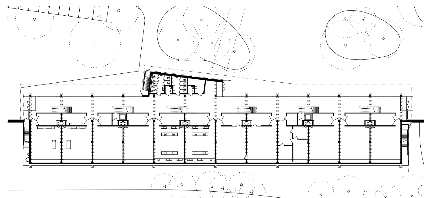
Erdgeschoss | Rez-de-chaussée
