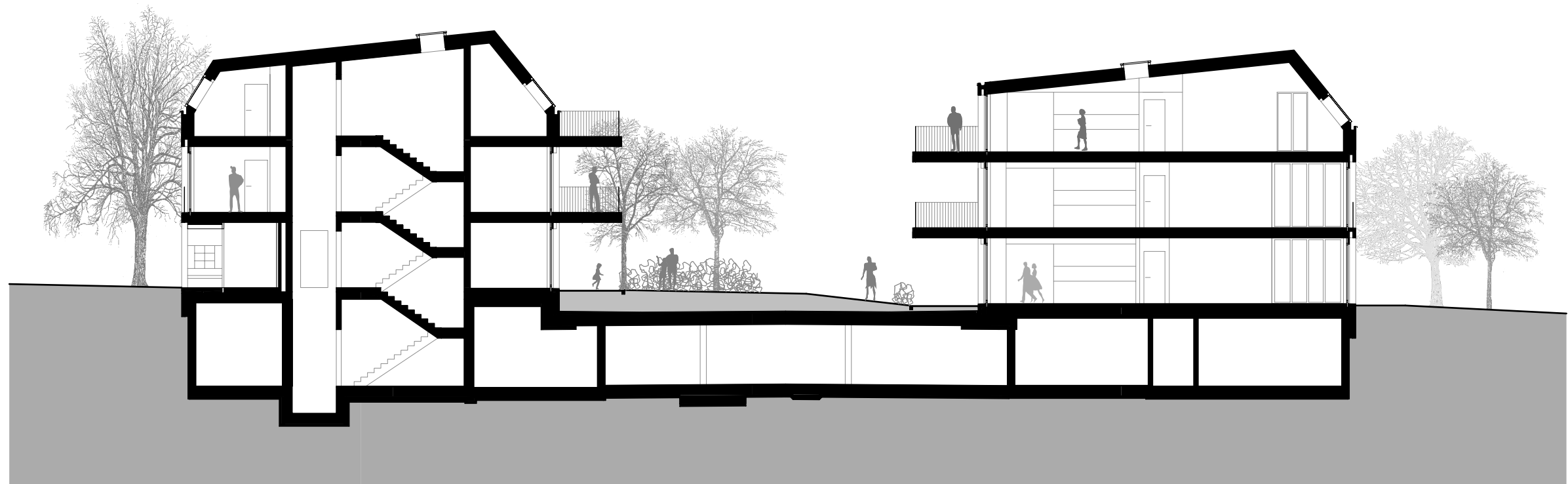
schnitt quer_haus bc
