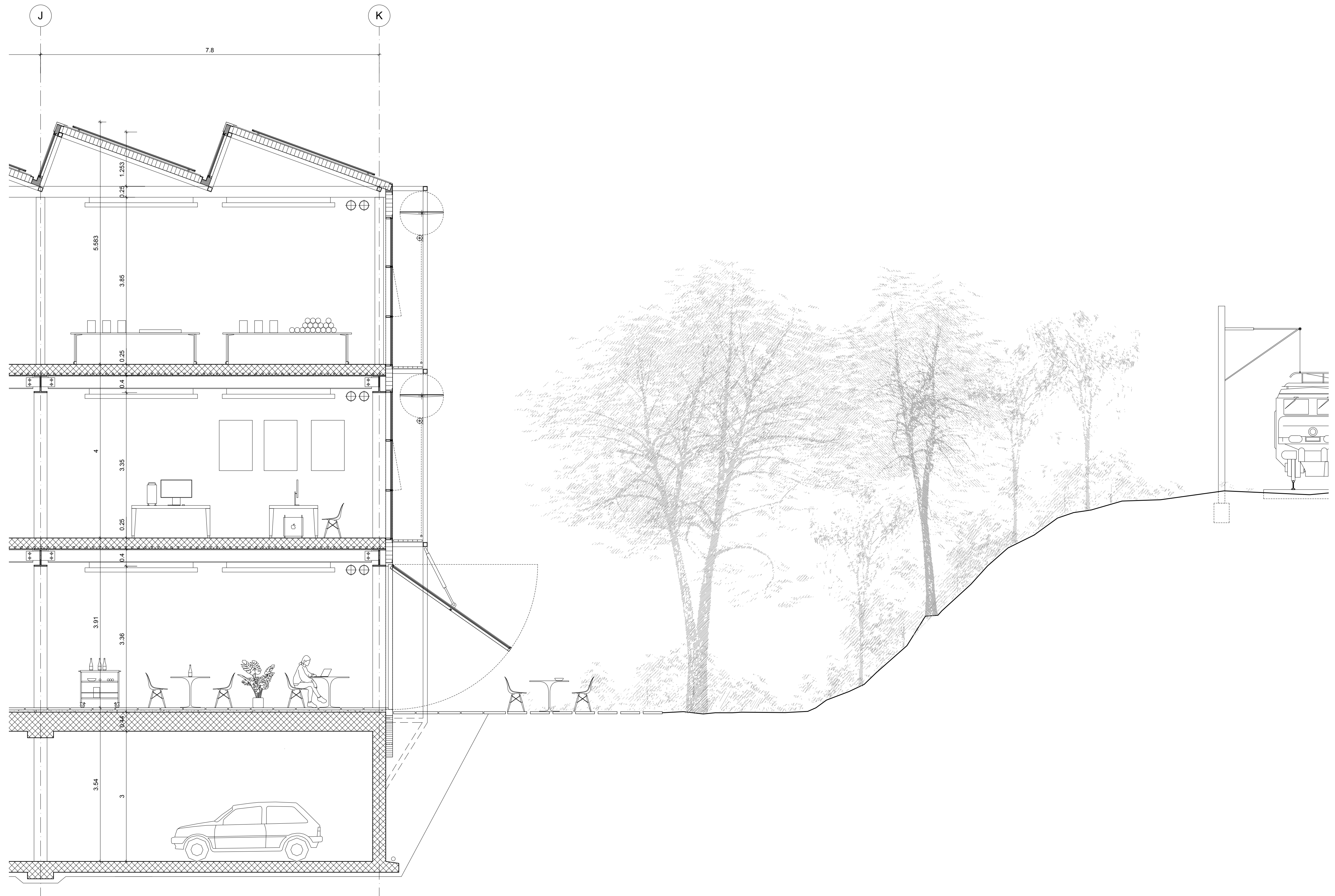
Coupe transversale - relation à l'axe ferroviaire Plug-In, 1:50
