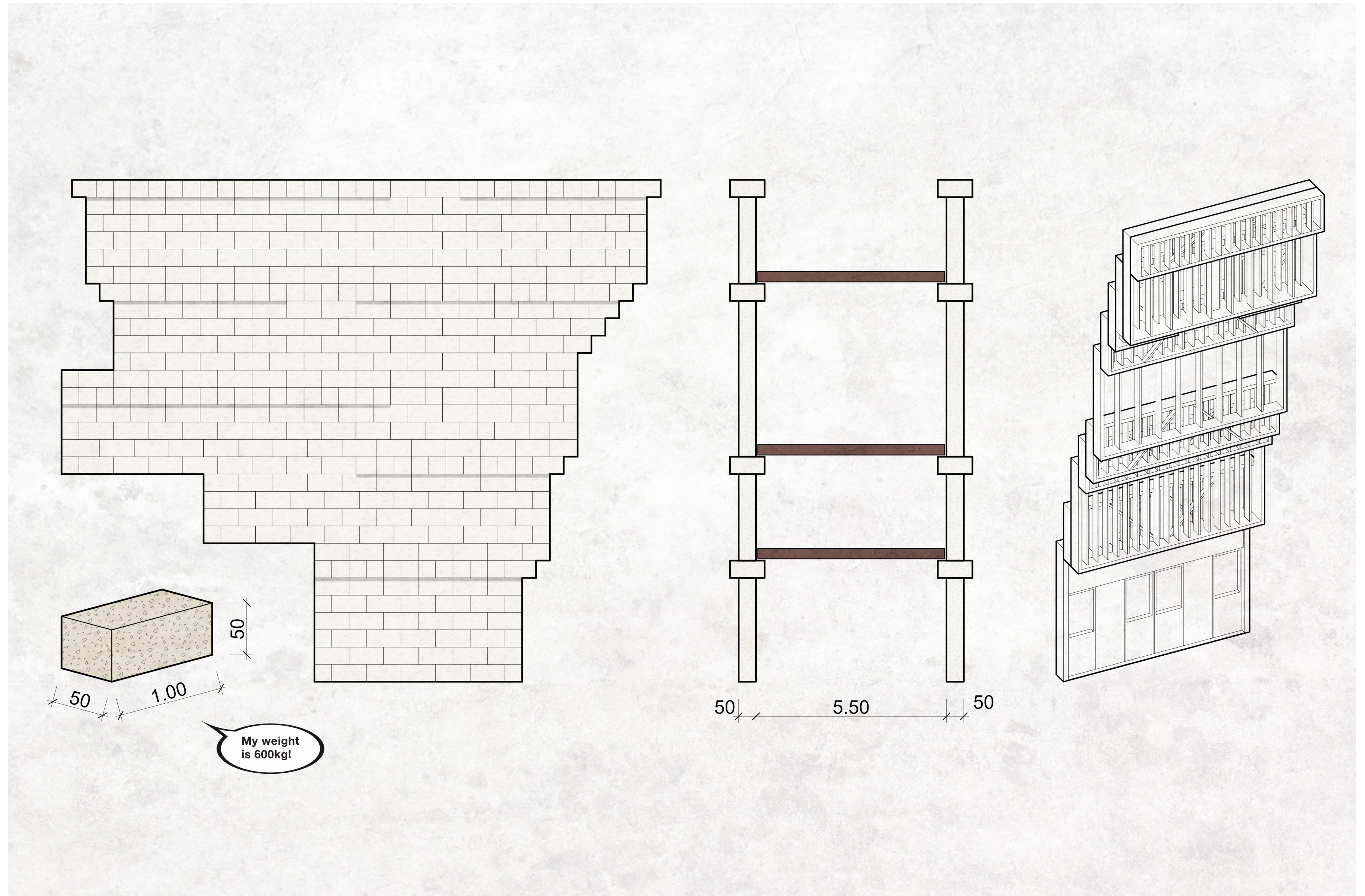
KONSTRUKTIONSPRINZIP WANDSCHOTTEN MIT HOLZFASSADE
