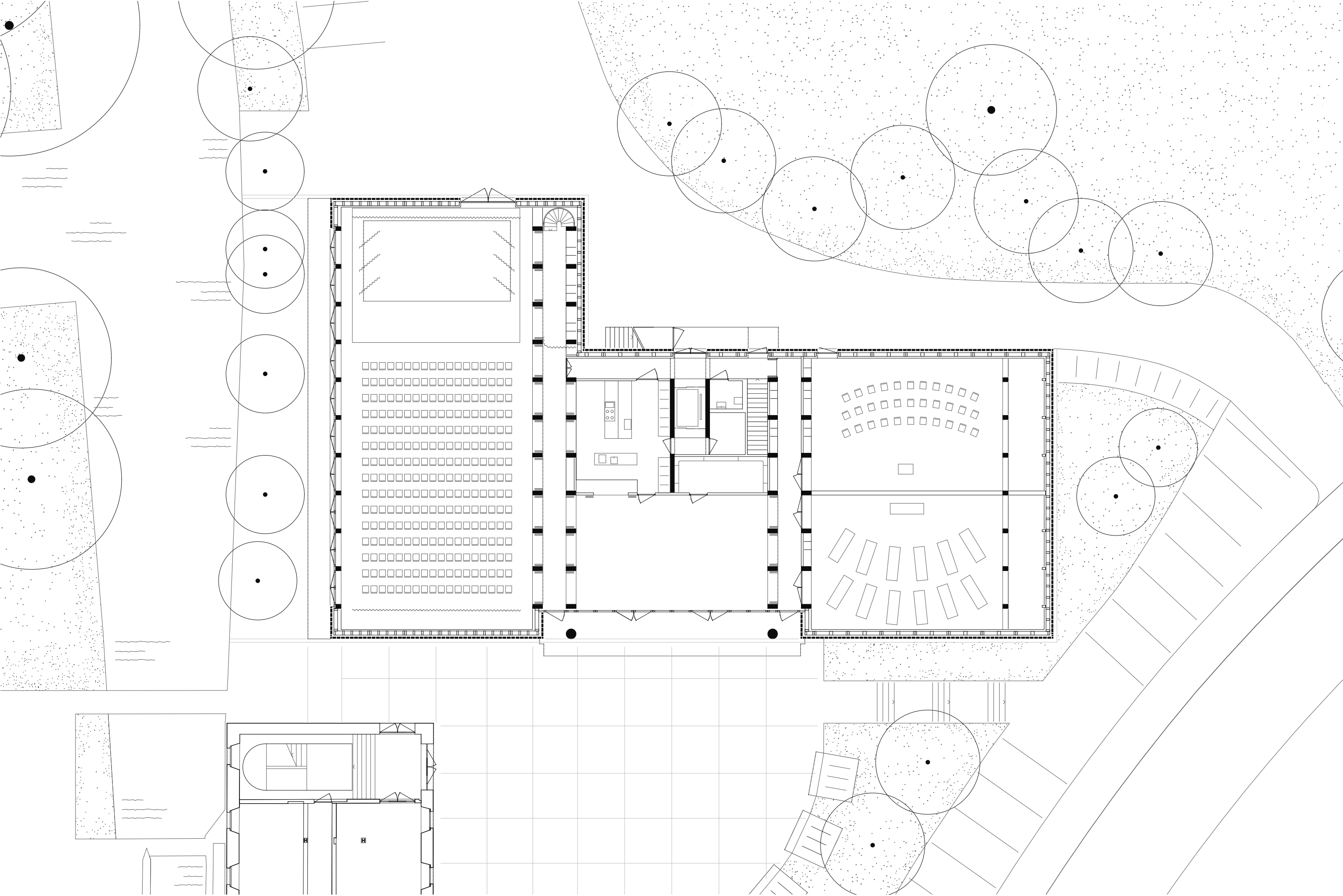
Grundriss Erdgeschoss 1:200
