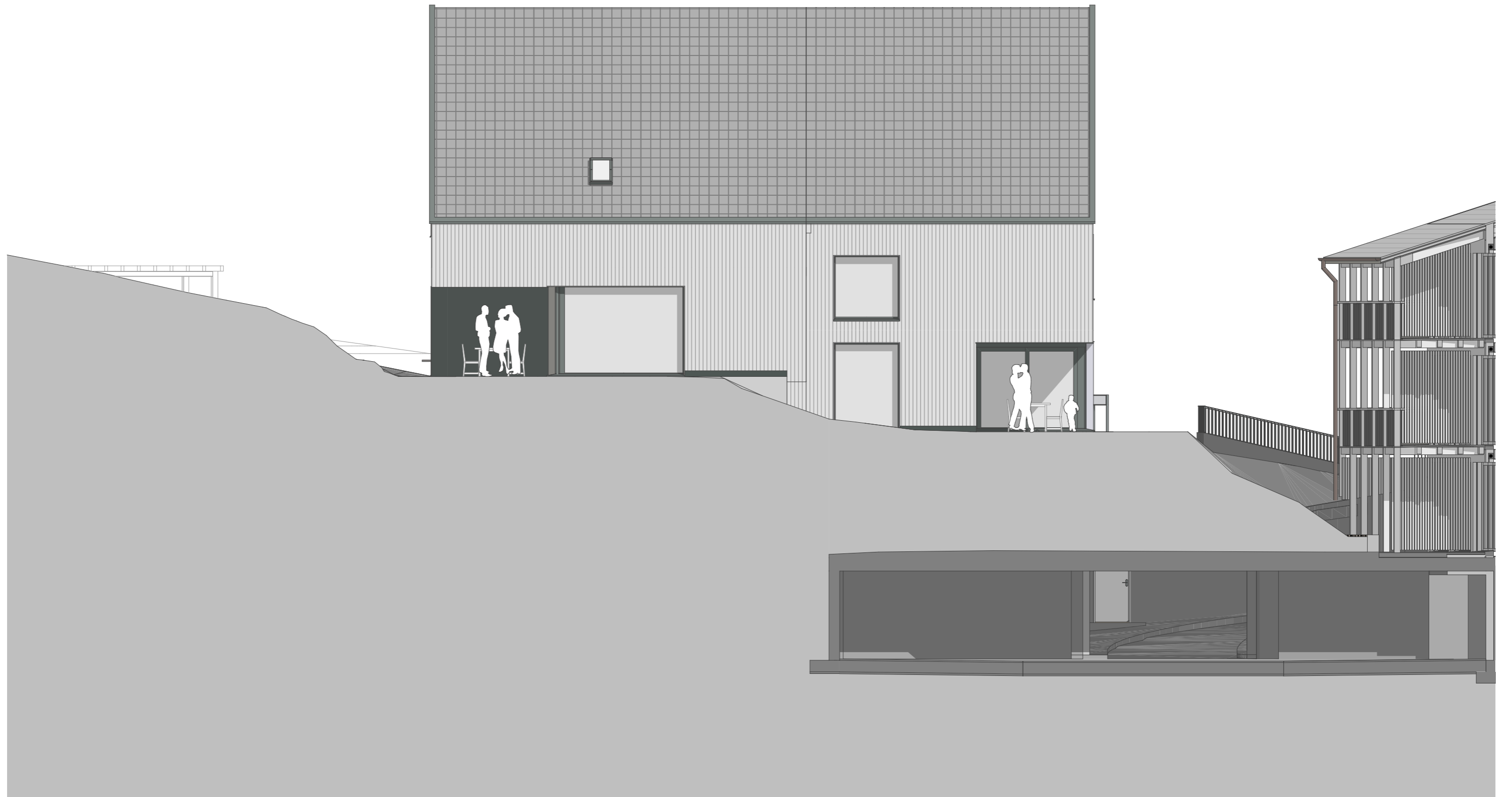
ANSICHT DEFH SÜD / 1:100
