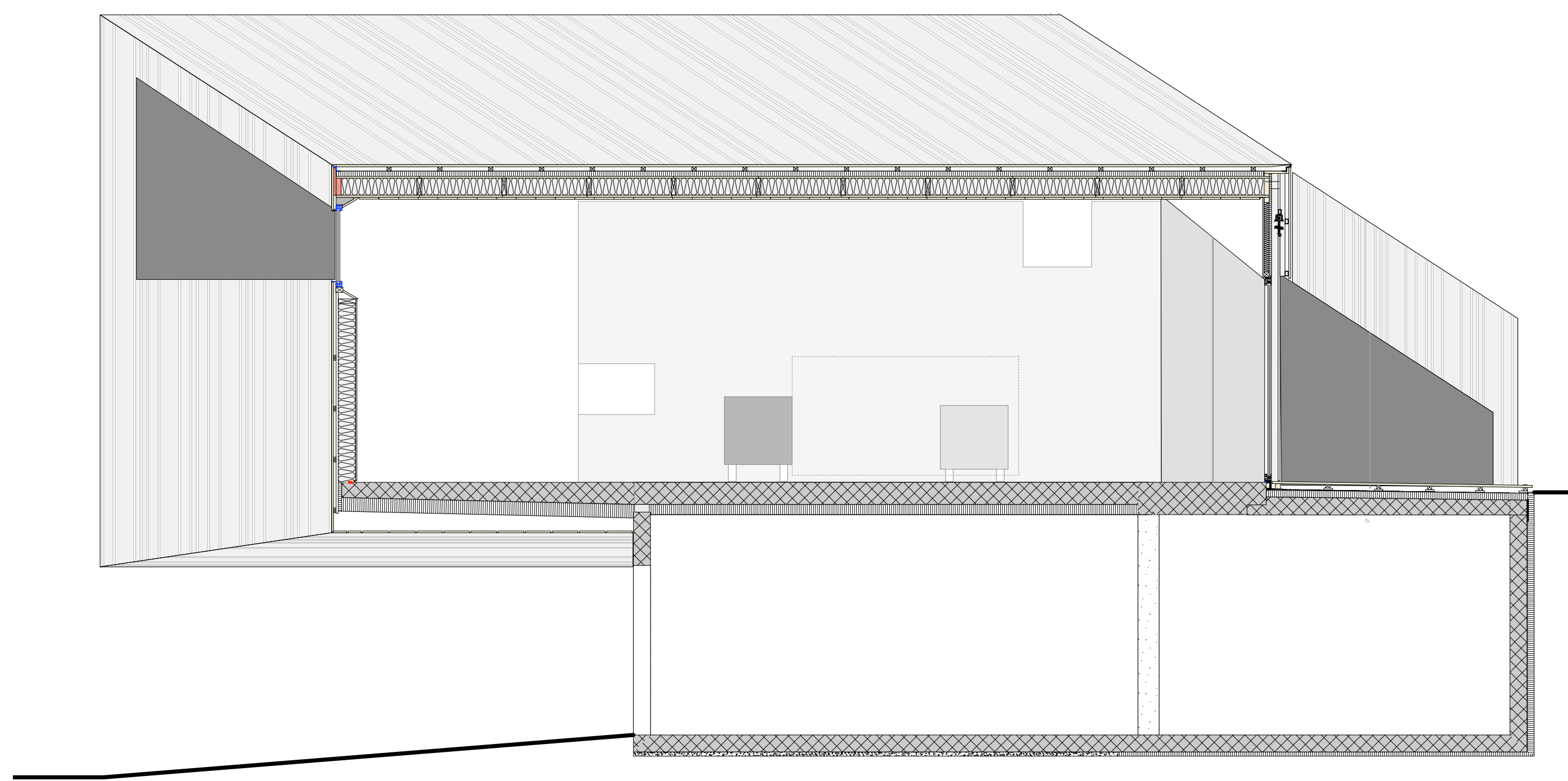
COUPE NORD-SUD
