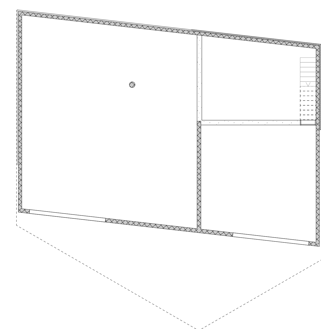
SOUS-SOL (1:100)
