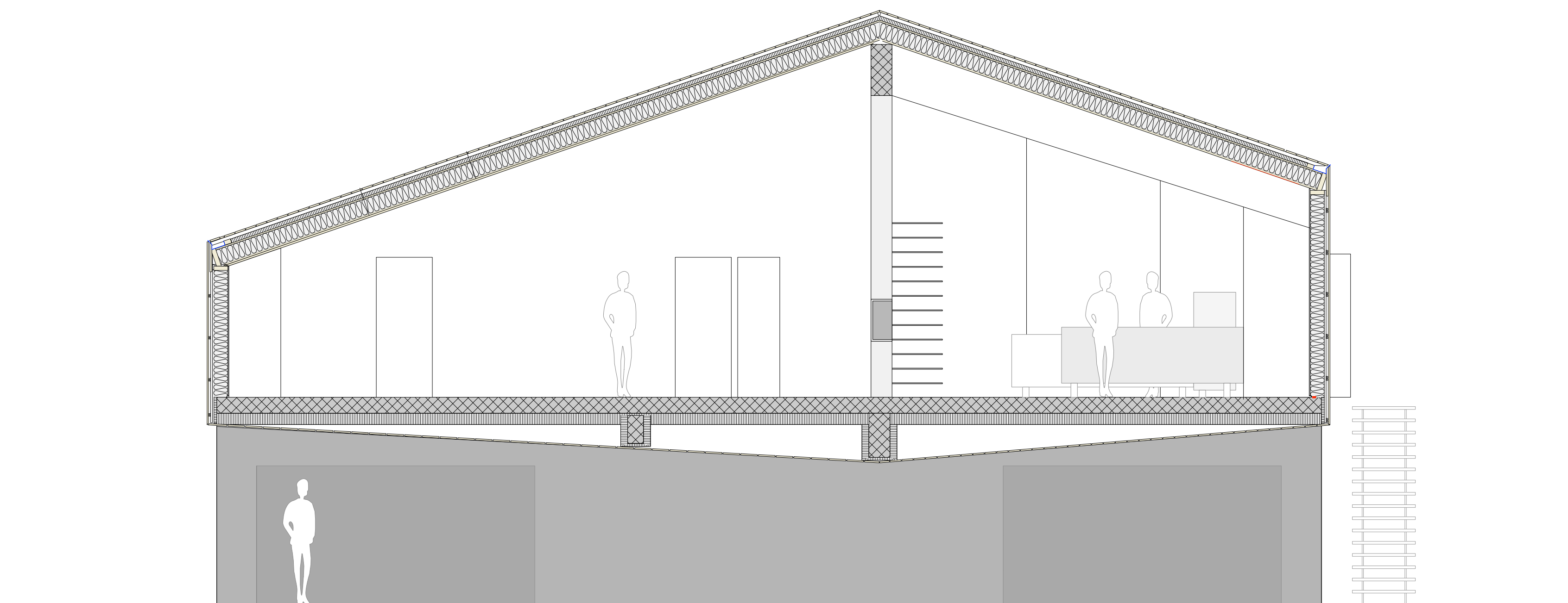
COUPE EST-OUEST
