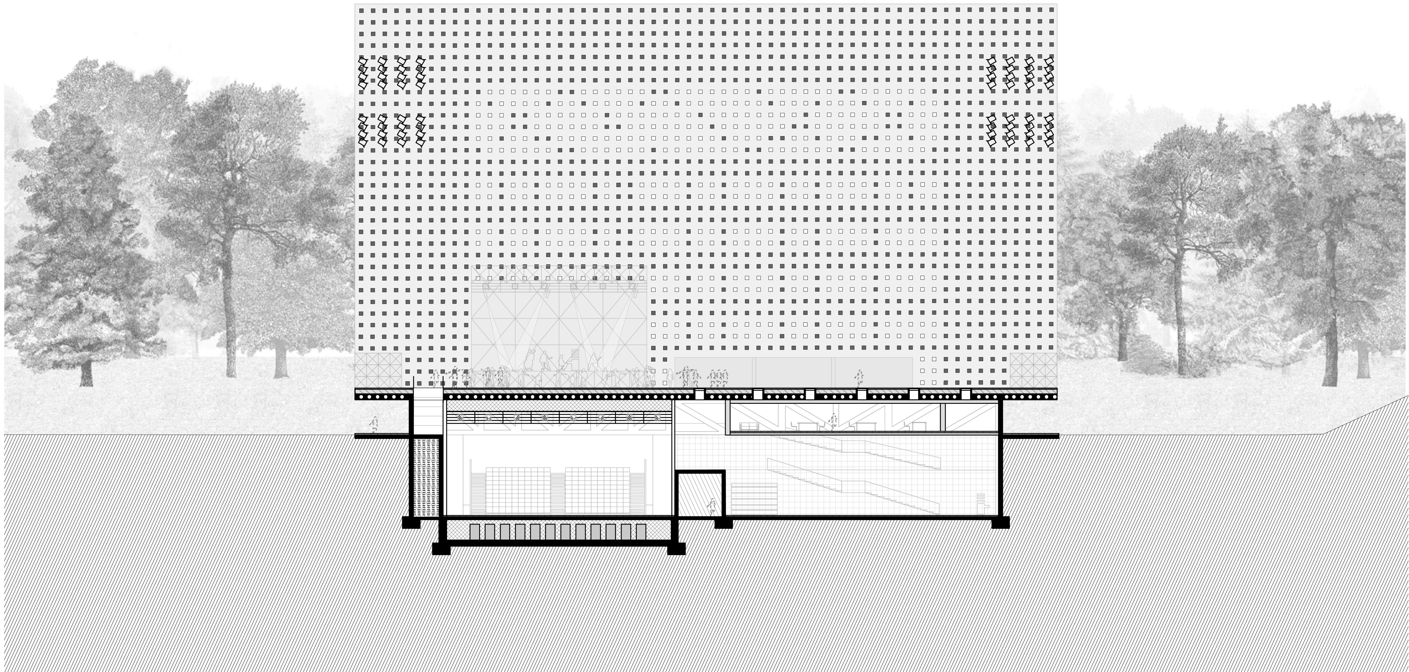
Schnitt cc
