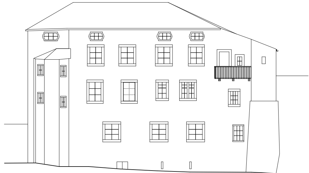
Westfassade 1:200
