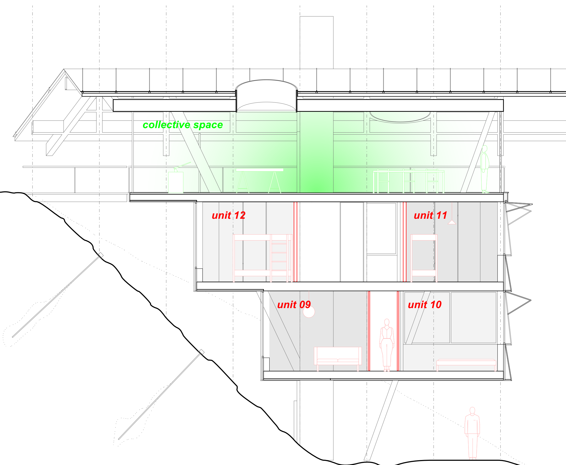
Querschnitt Sommer
