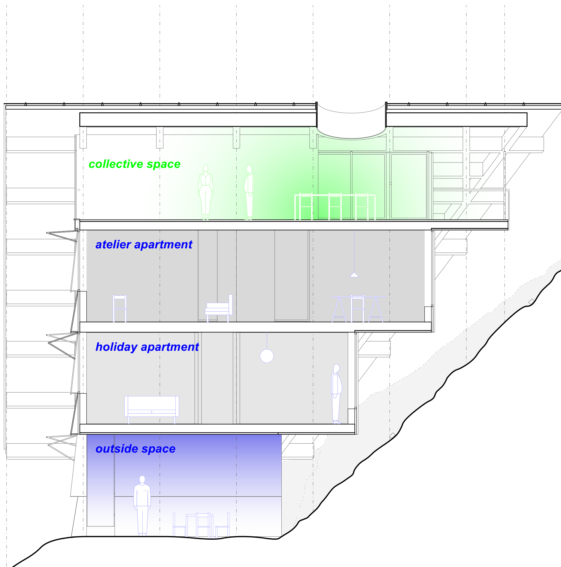
Querschnitt Sommer
