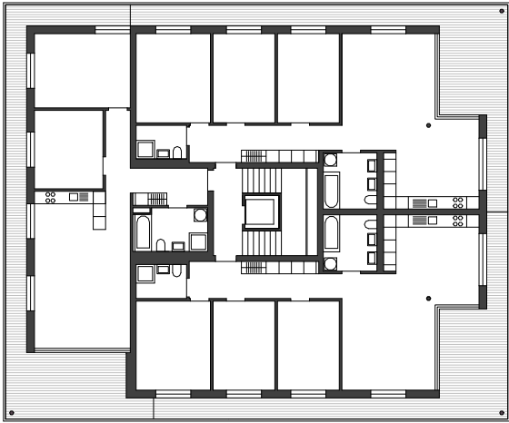
1./2./3. Obergeschoss
