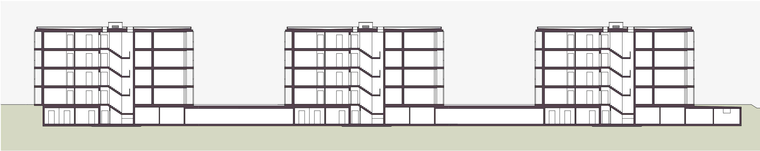
Längsschnitt
