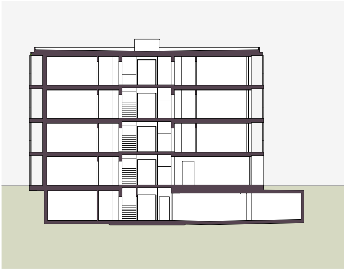
Querschnitt
