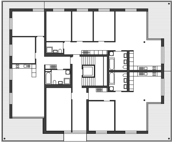
Erdgeschoss
