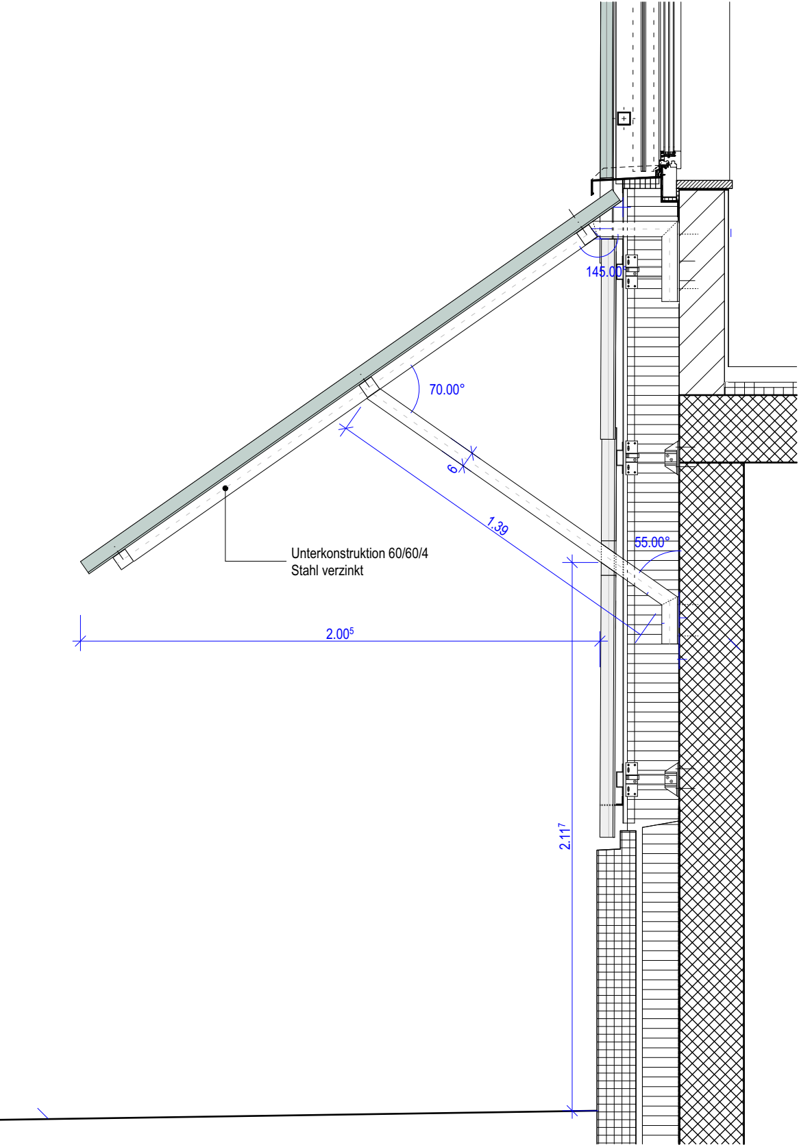
Schnitt A
