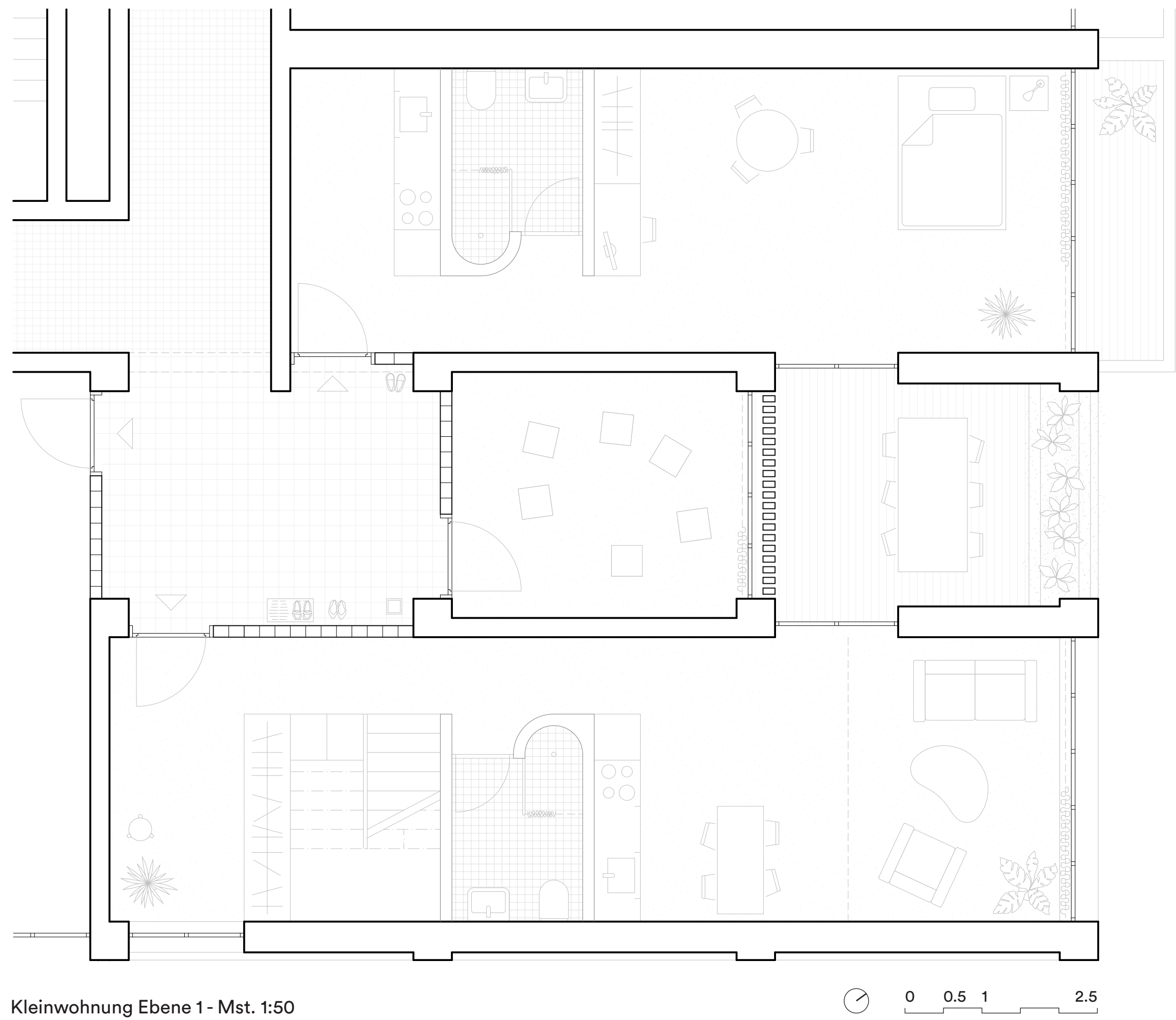
Kleinwohnung Ebene 1 - Mst. 1:50
