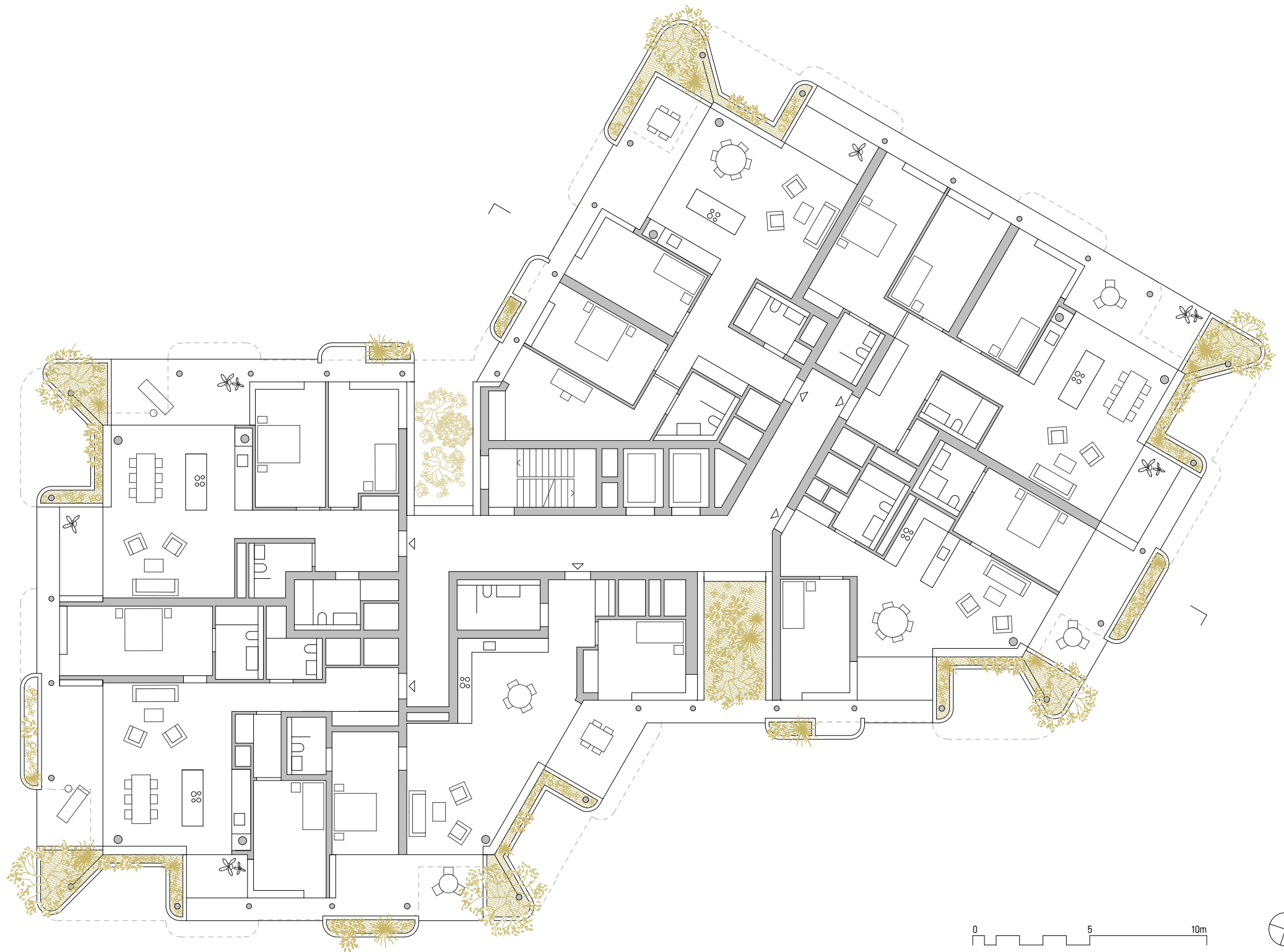
Gartenhochhaus Aglaya 12. Obergeschoss
