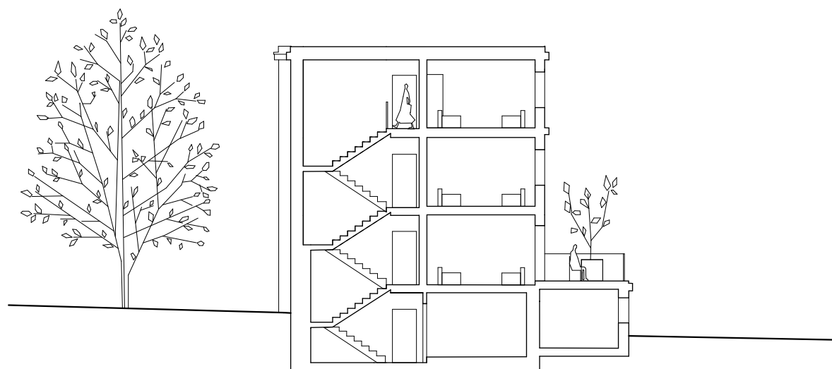
COUPE BB 1/200
