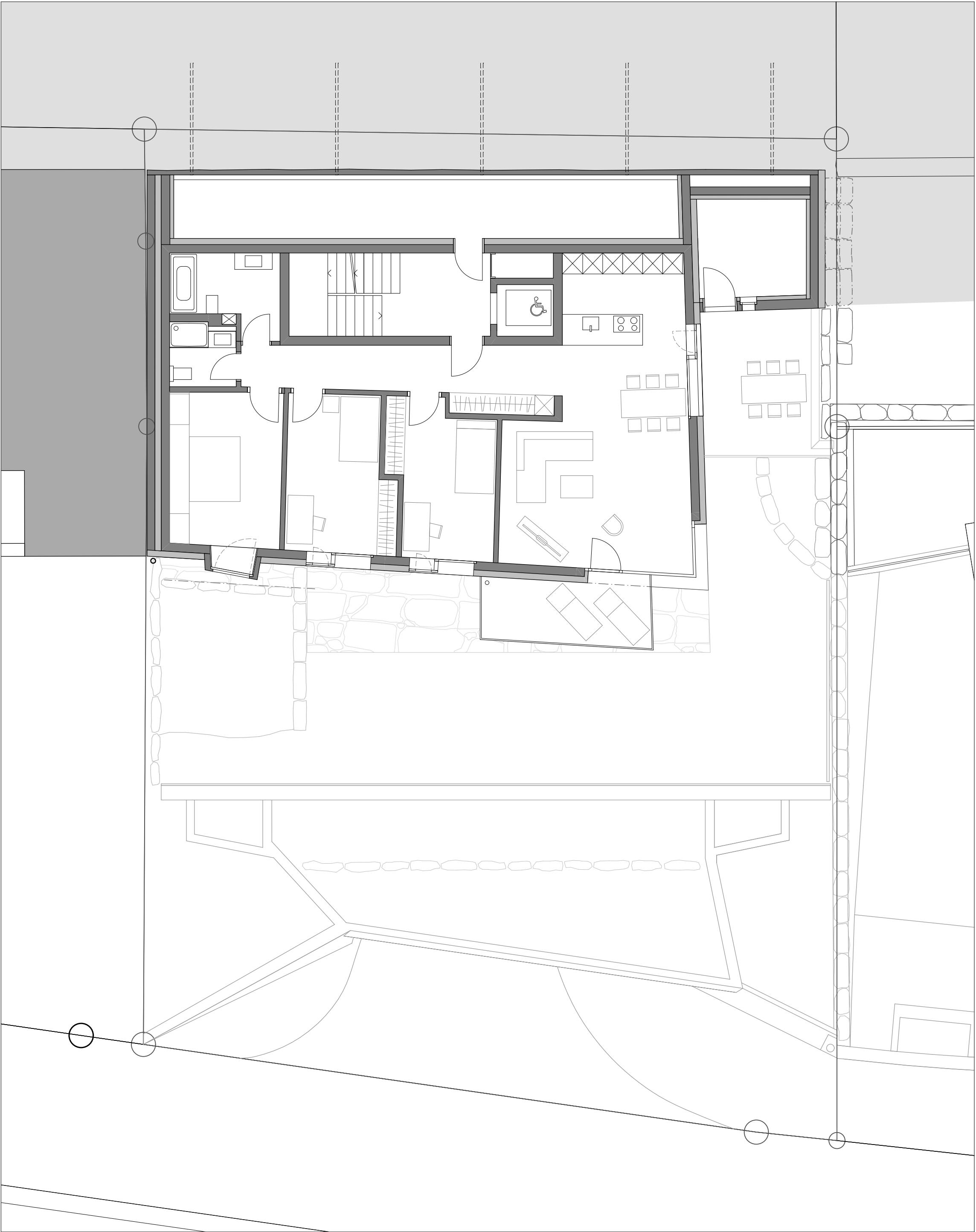
GRUNDRISS 2. OBERGESCHOSS
