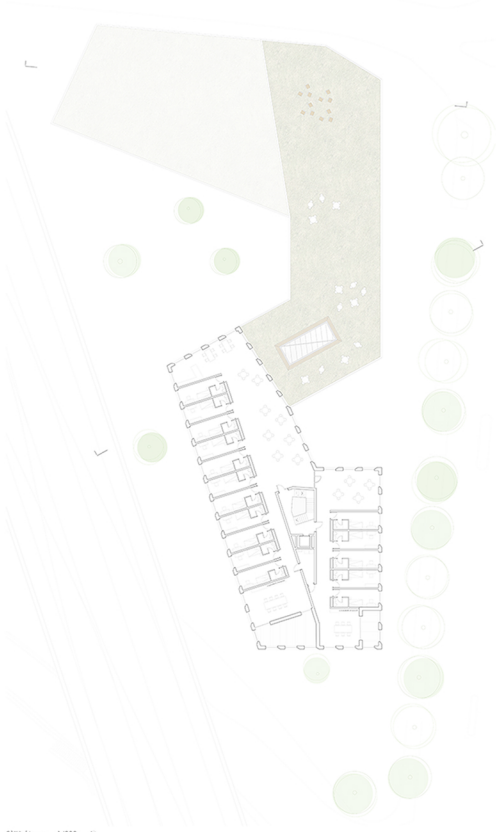
3 rd étage - 1/200
