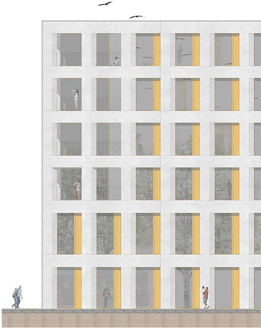
Façade - 1/50
