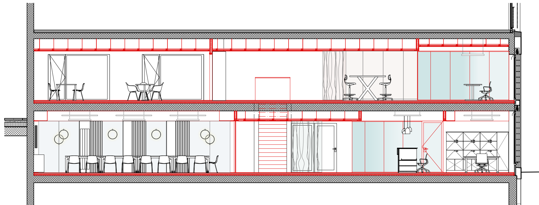
Coupe A-A
