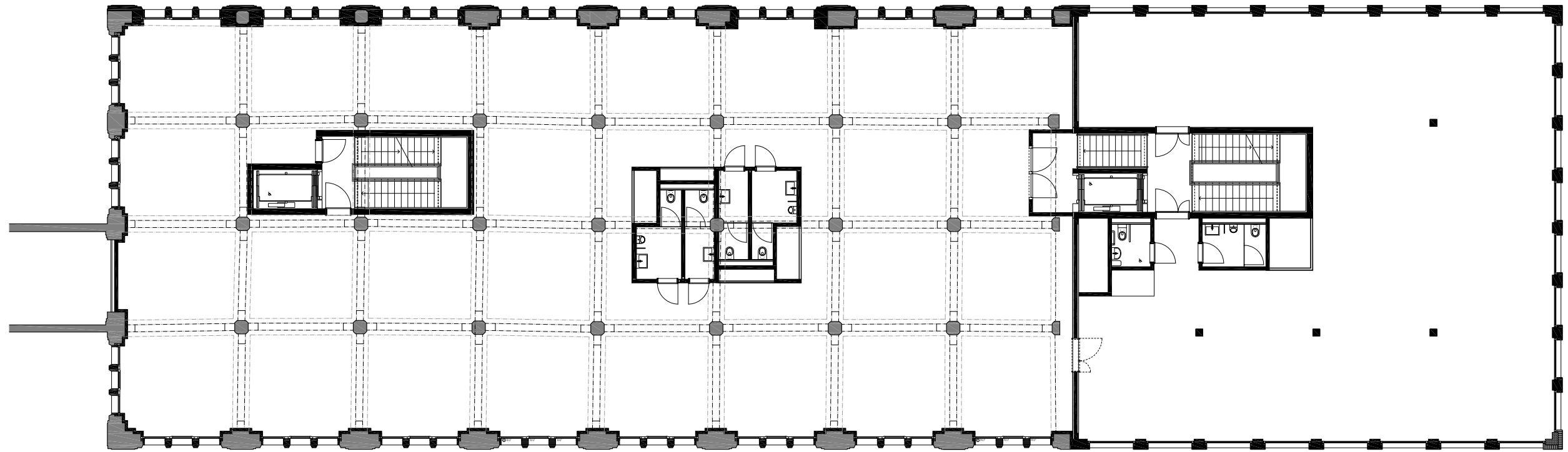
Regelgeschoss
