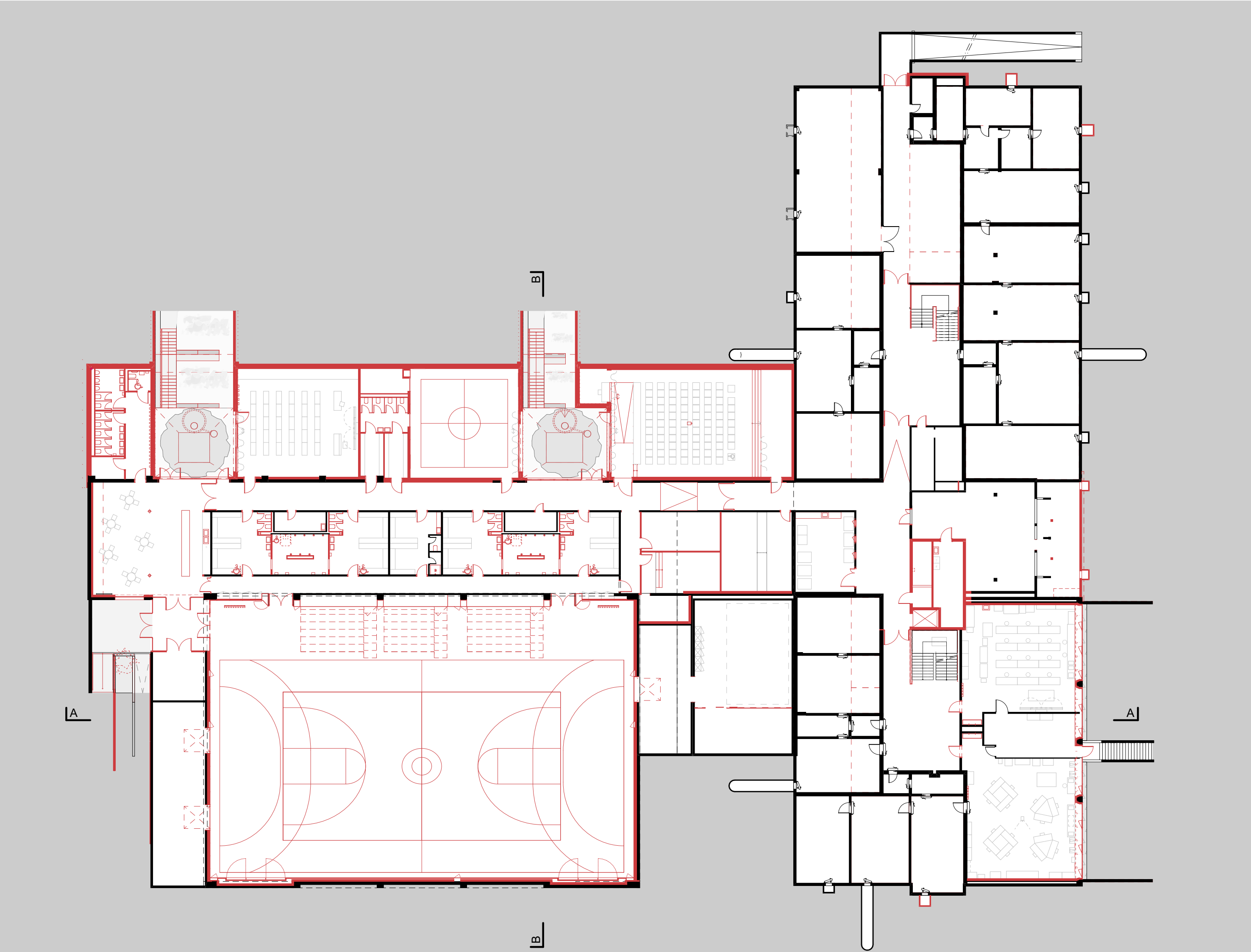
Plan sous-sol - 1:300
