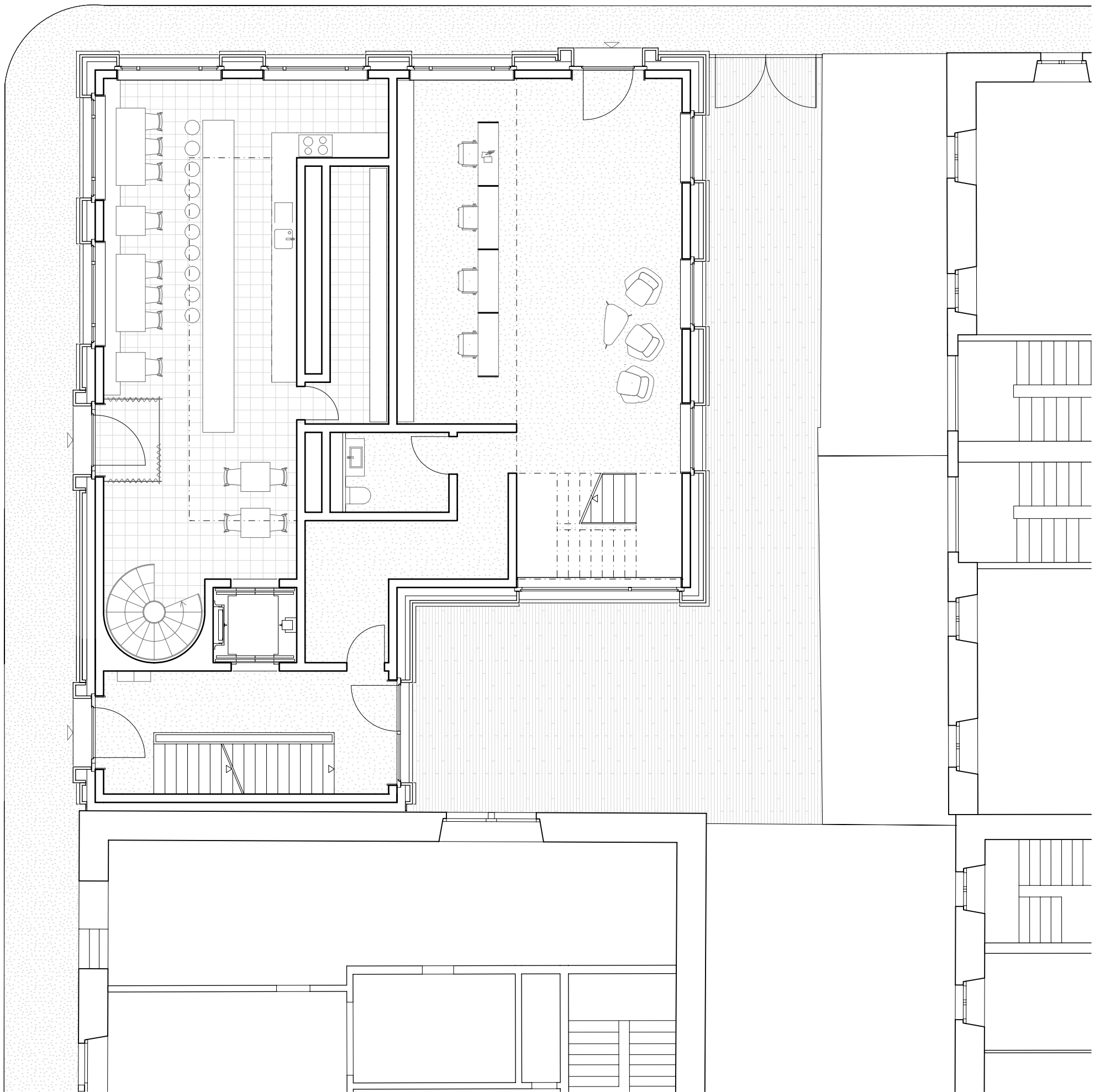
Grundriss EG 1:100
