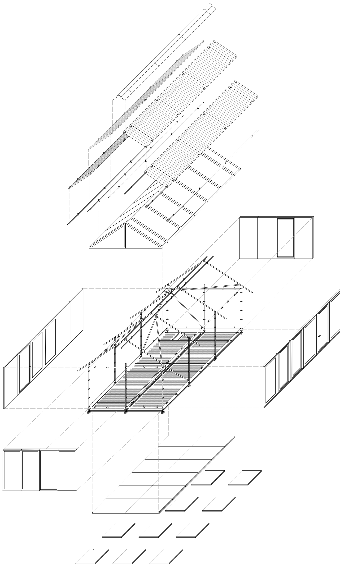
EXPLOSIONSZEICHNUNG
