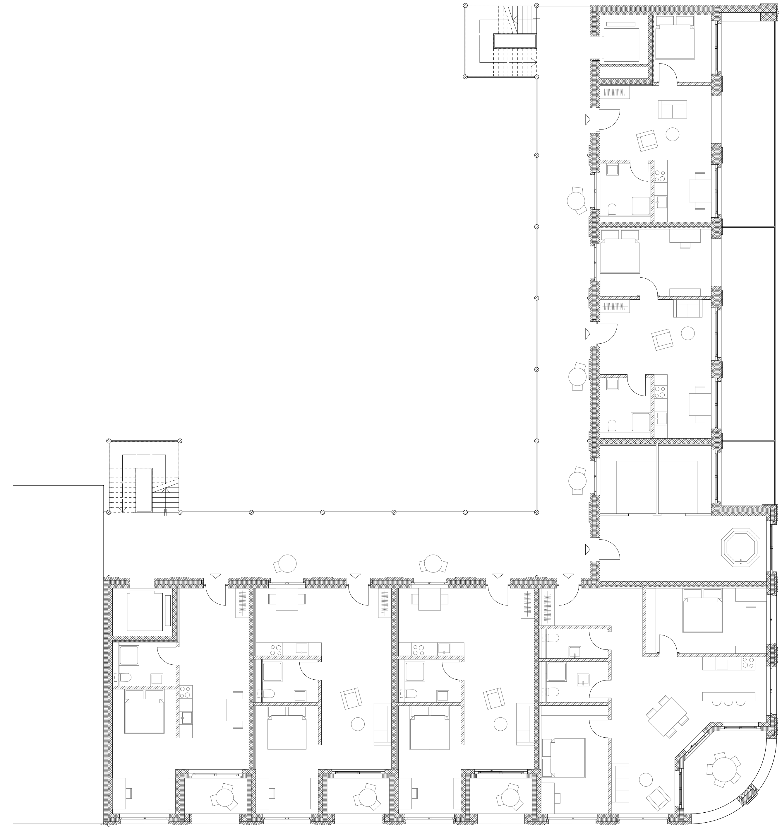
GRUNDRISS 4.OG, 1:100
