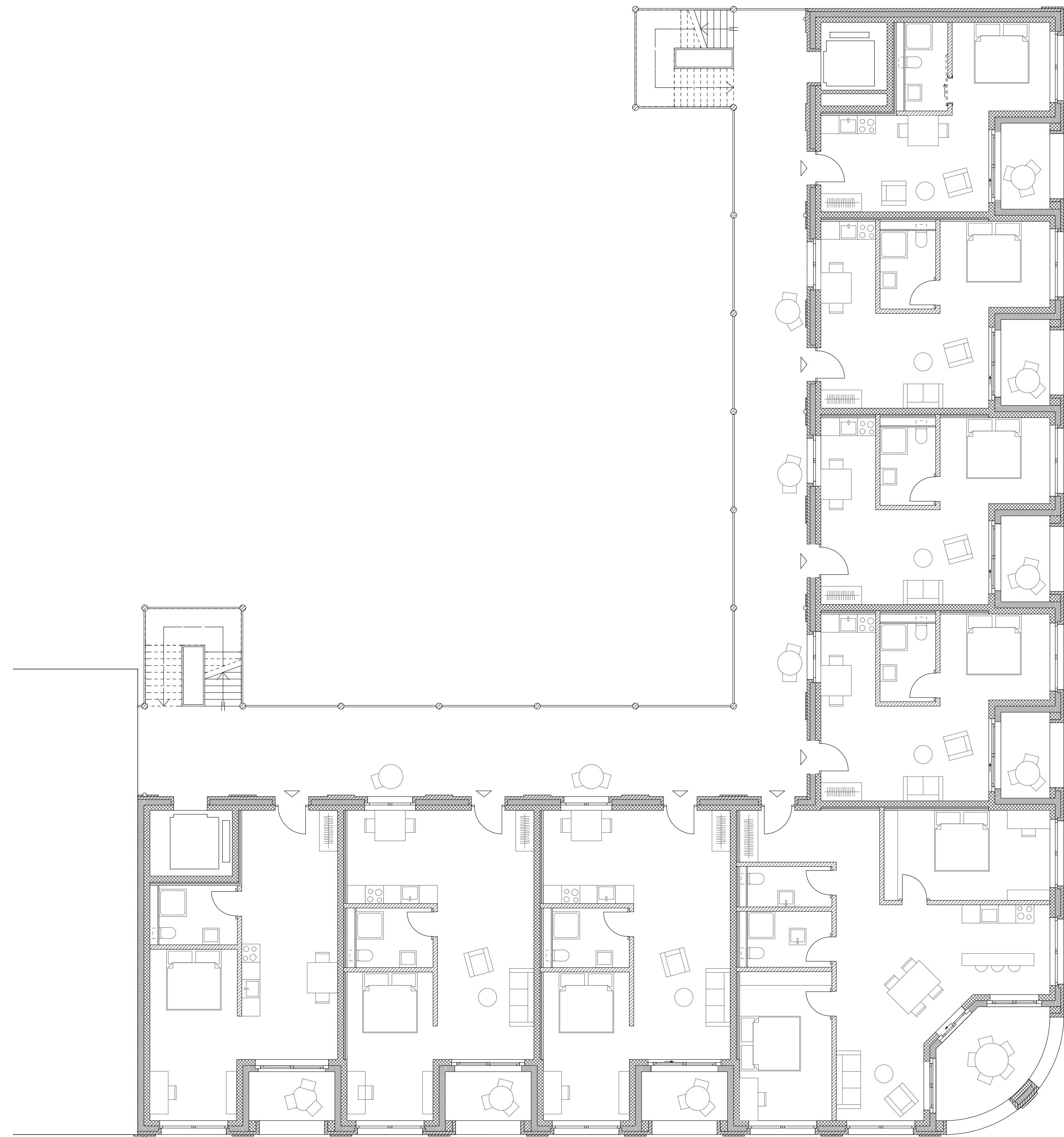
GRUNDRISS 1.-3.OG, 1:100
