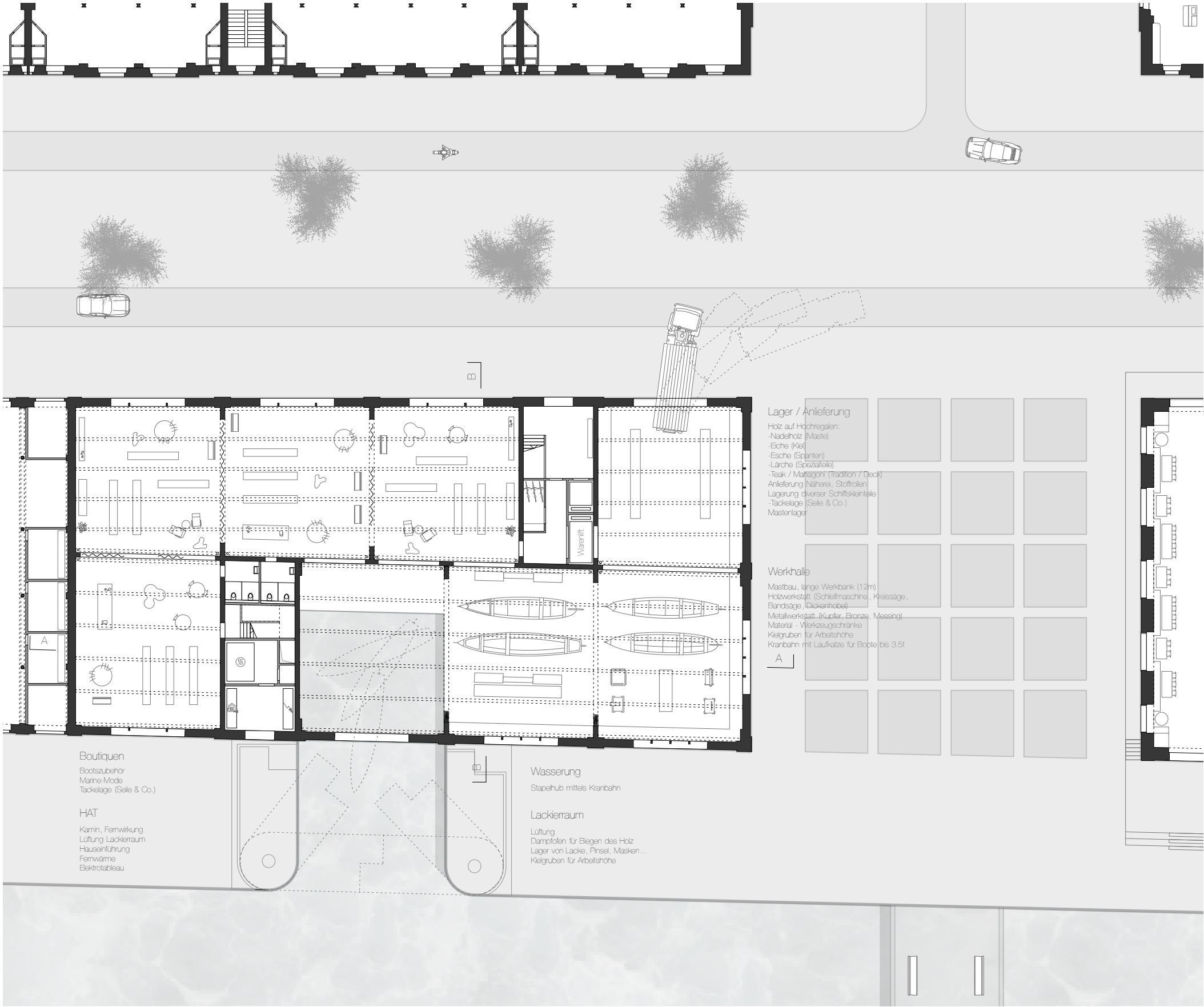
Grundriss Erdgeschoss
