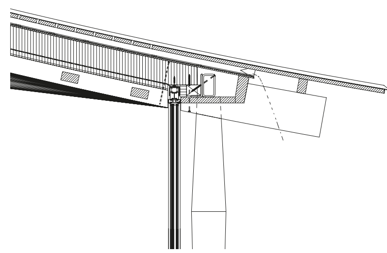
Detail Vordach Traufe:
