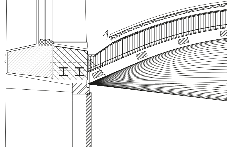
Detail Dachaufbau:
