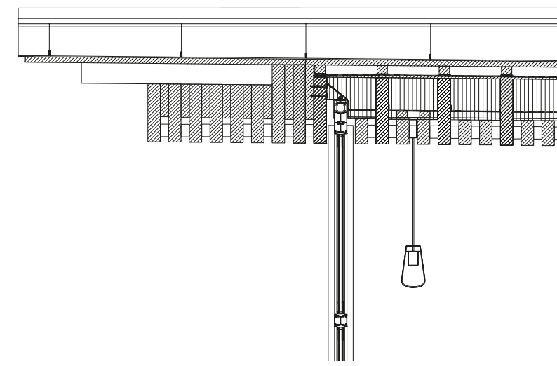
Detail Vordach Ortgang:
