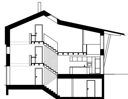
Schnitt A | Coupe A
