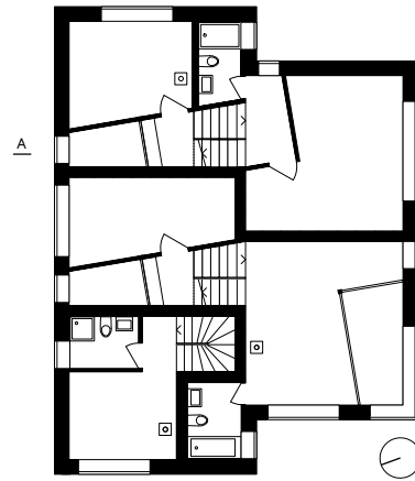
Erdgeschoss | Rez-de-chaussée
