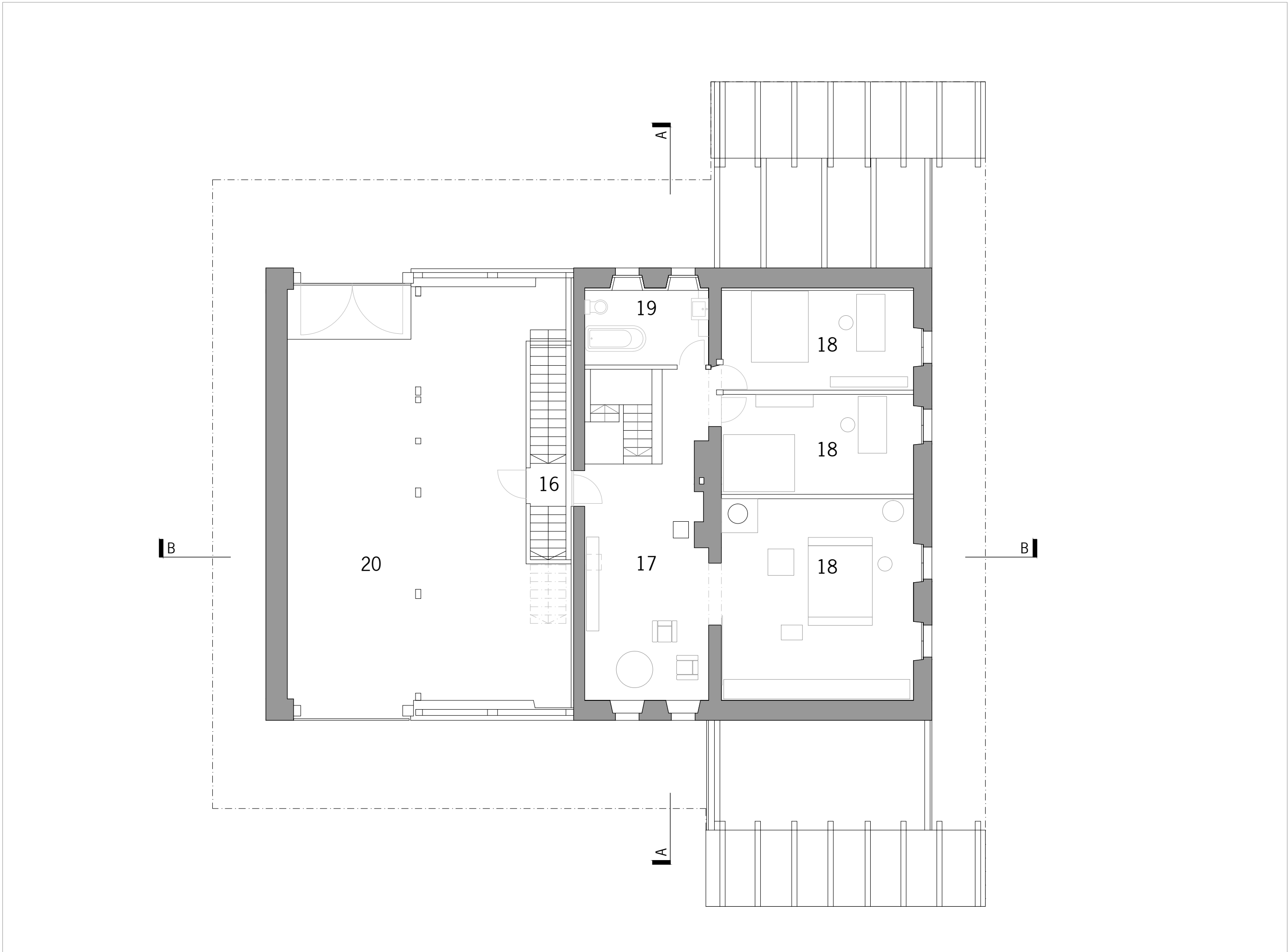
obergeschoss/étage supérieur
