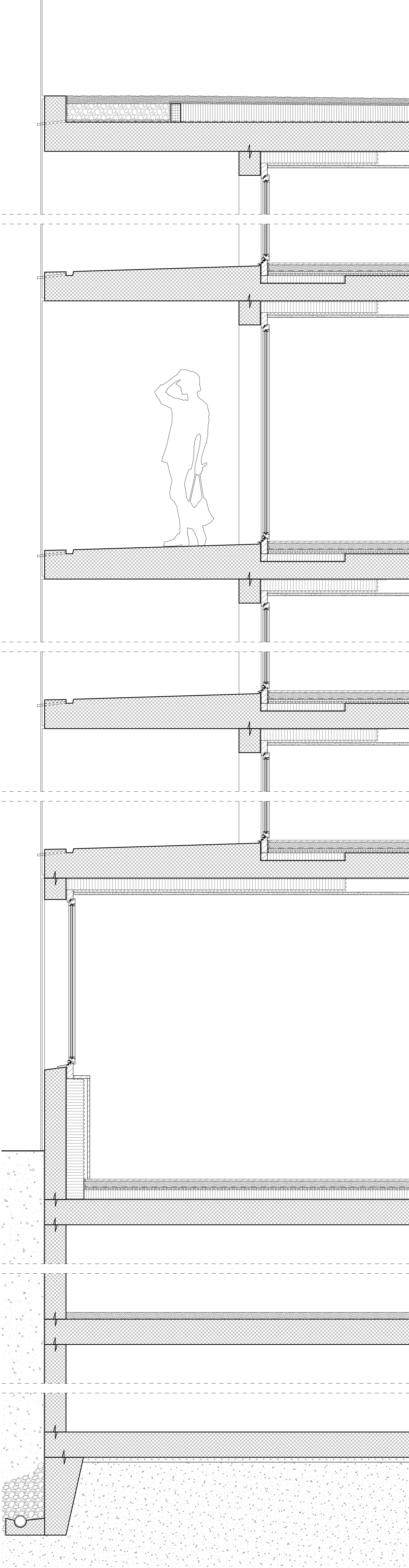
Travée coursives 1:20
