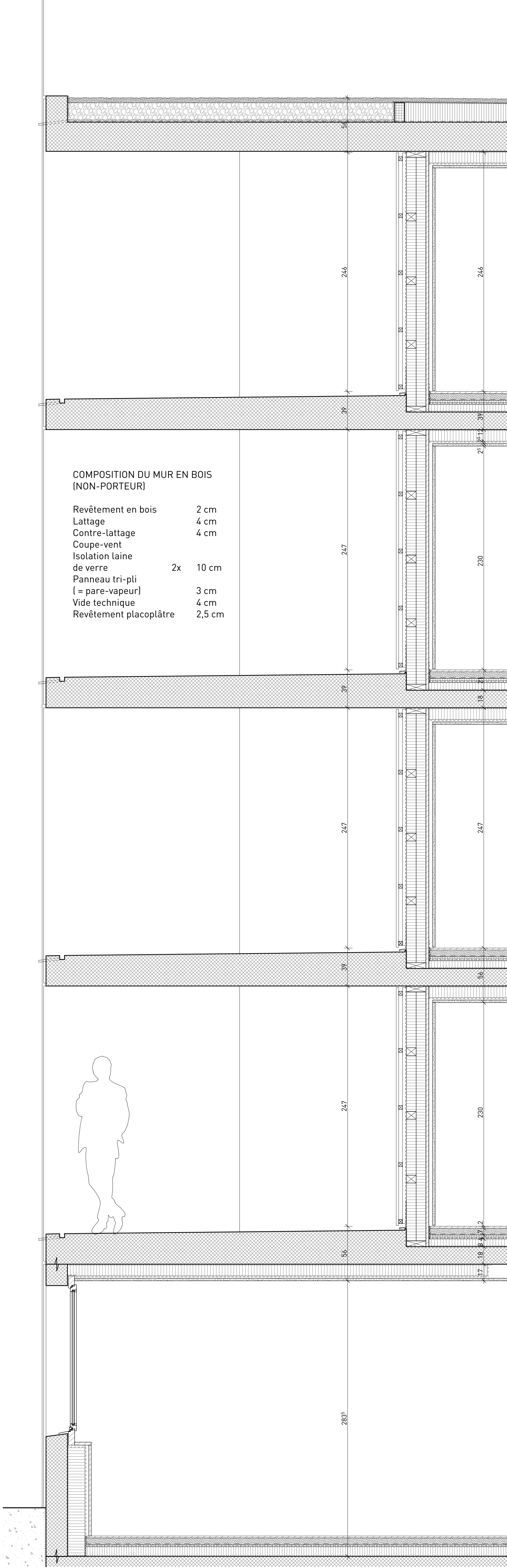
Travée coursives 1:20
