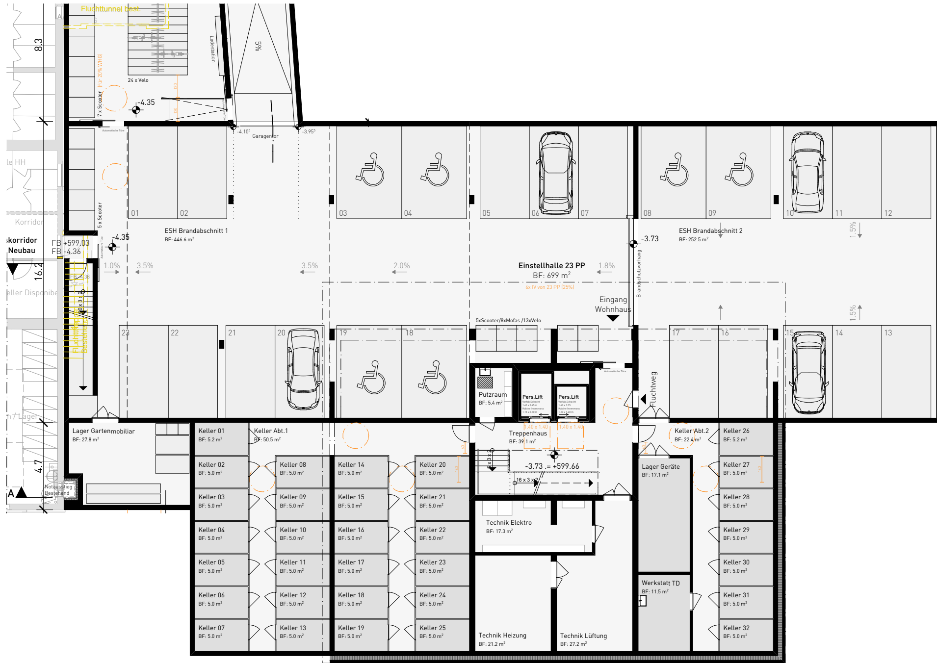
Haus am Mühlbach, Alterssiedlung Bodmer, Chur Baudokumentation | Grundriss 1.UG
