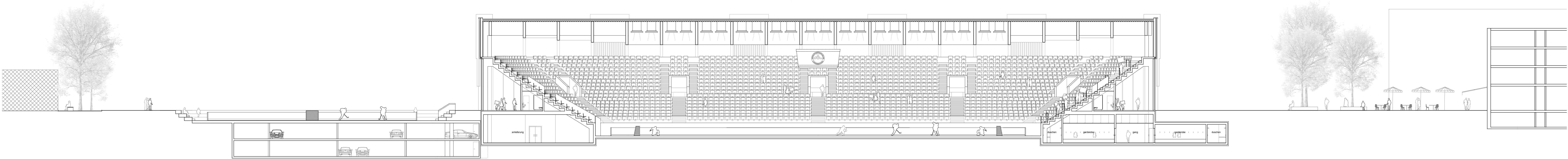
langsschnitt a-a 1:200
