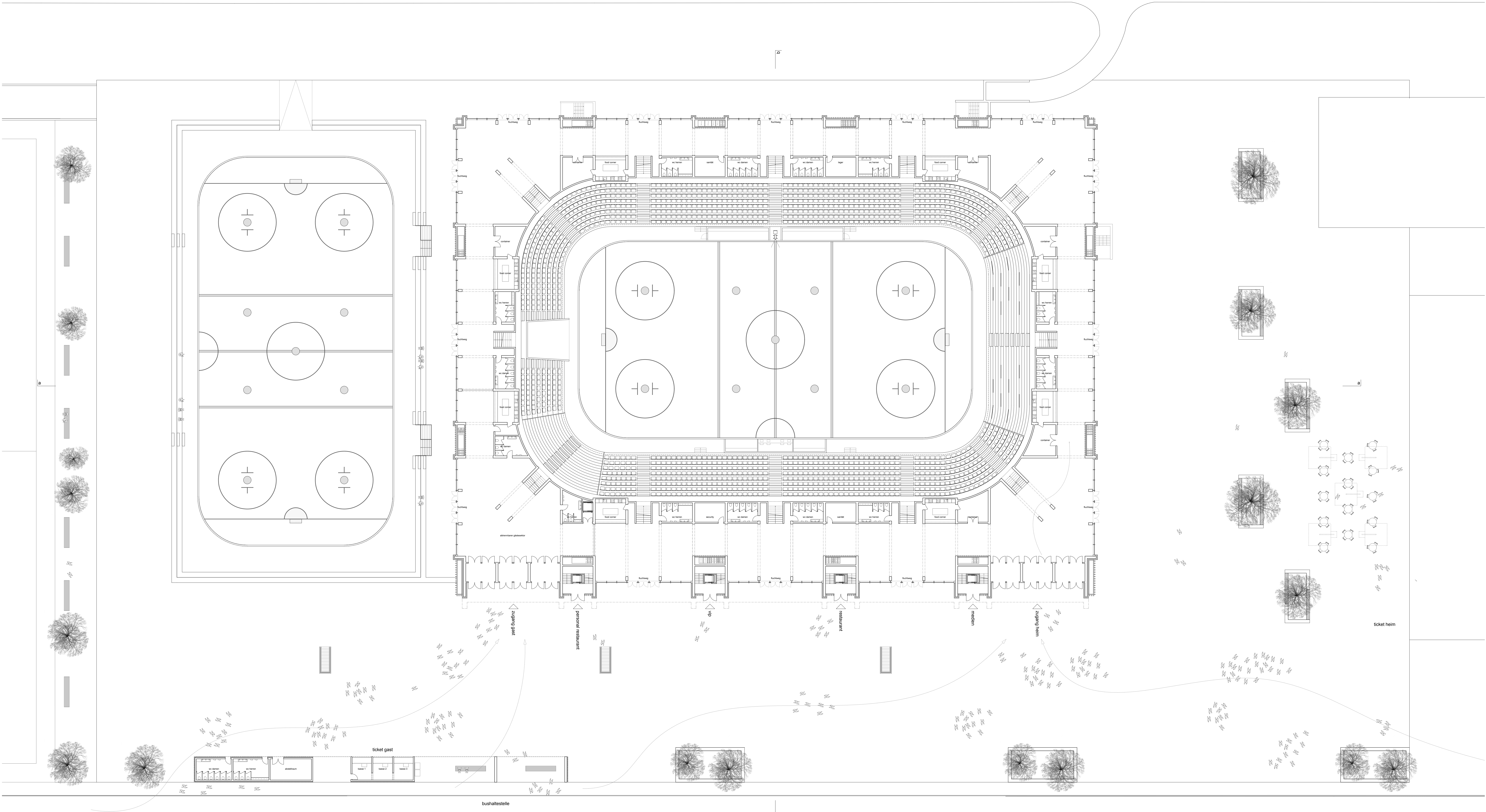
erdgeschoss 1:200
